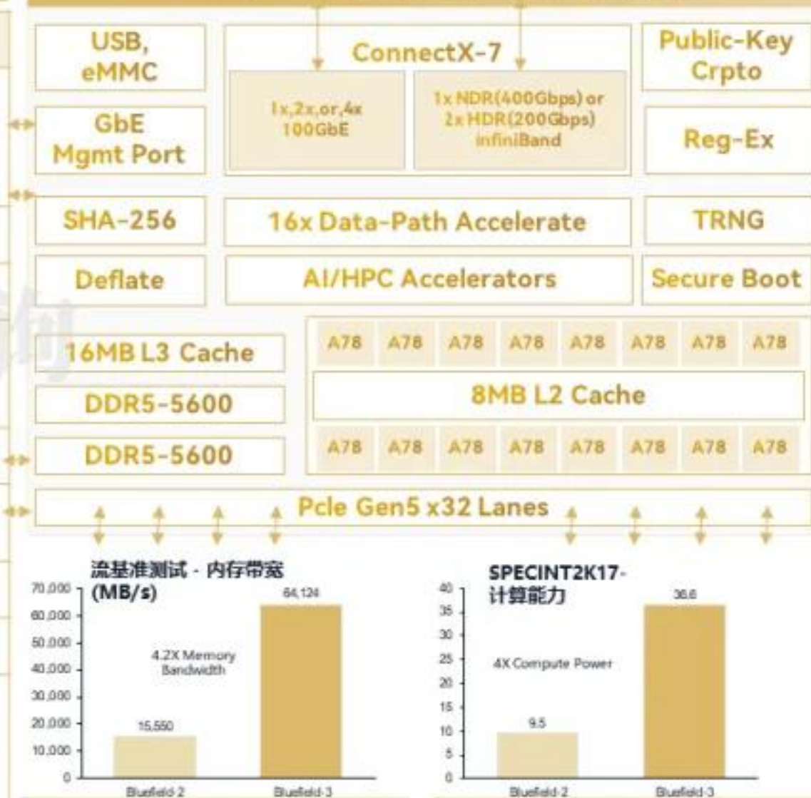
图1. 与NVIDIA BlueField-2 DPU 相比, NVIDIA BlueField-3 DPU 的内存带宽和计算能力提高了四倍
