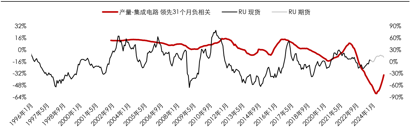
图表 278: 集成电路产量 M+31指数
