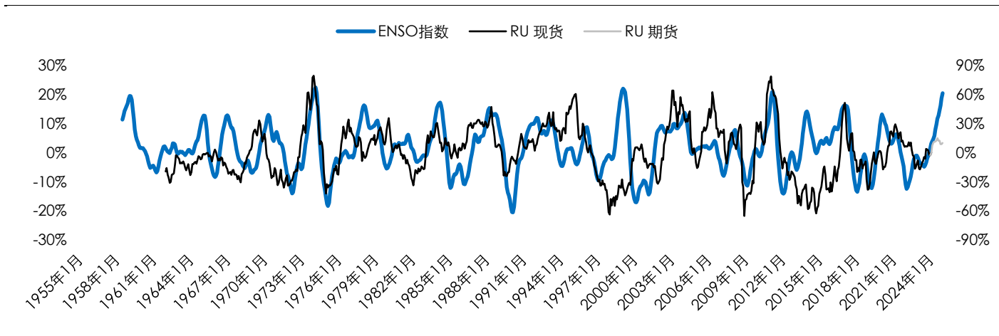
图表 5： ENSO M+15指数
