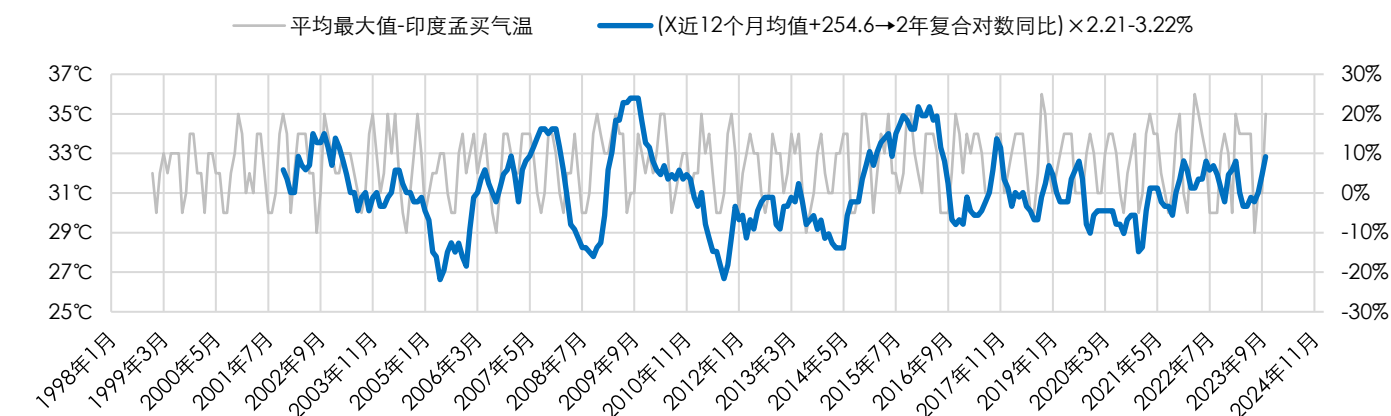
图表 15: 平均最大值-印度孟买气温
