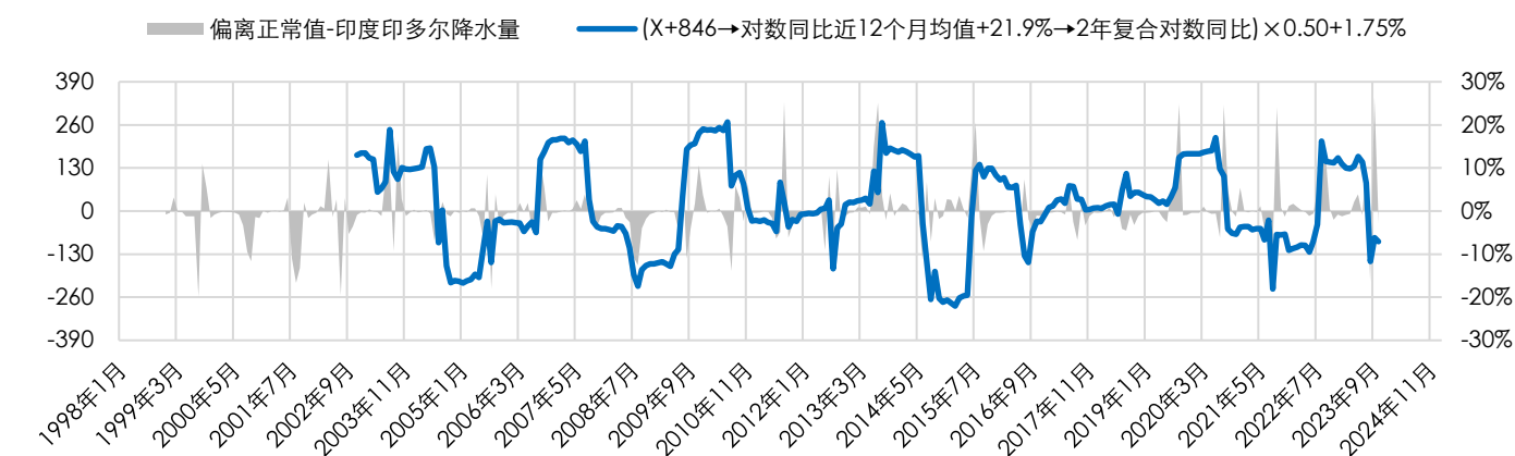
图表 17：偏离正常值-印度印多尔降水量 (mm)
