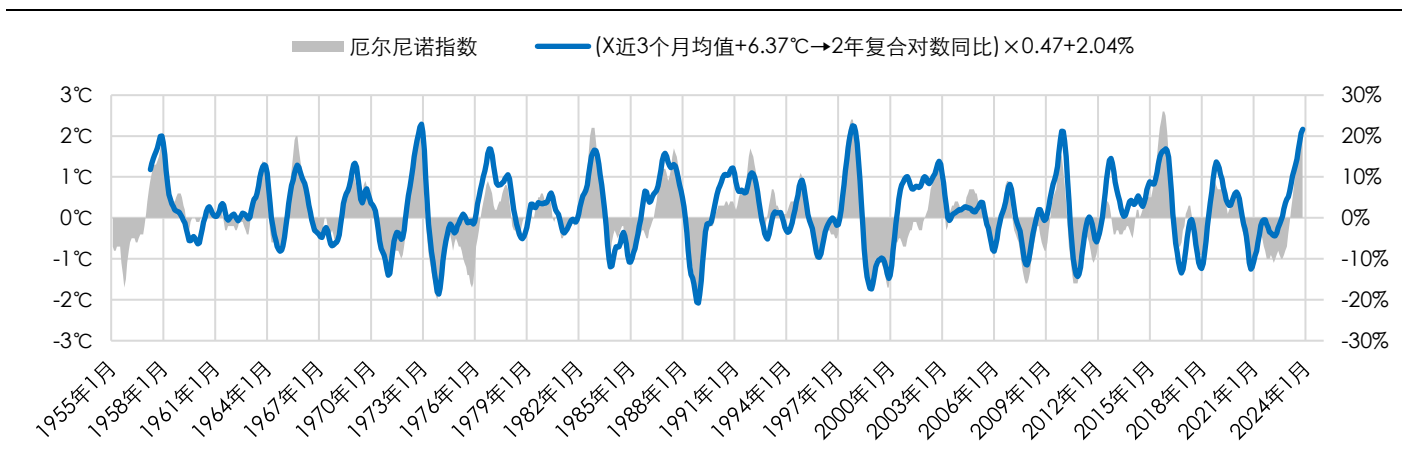
图表 6： NINO 3.4指数
