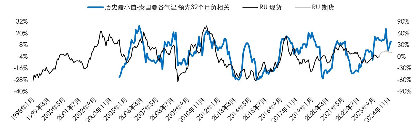
图表 14: 历史最小值-泰国曼谷气温 M+32指数
