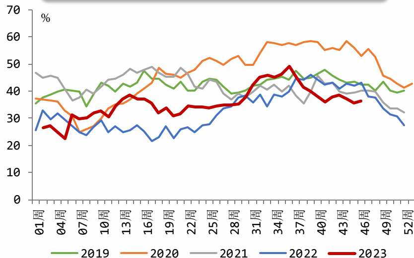
四季度石油沥青装置开工率触底回升
