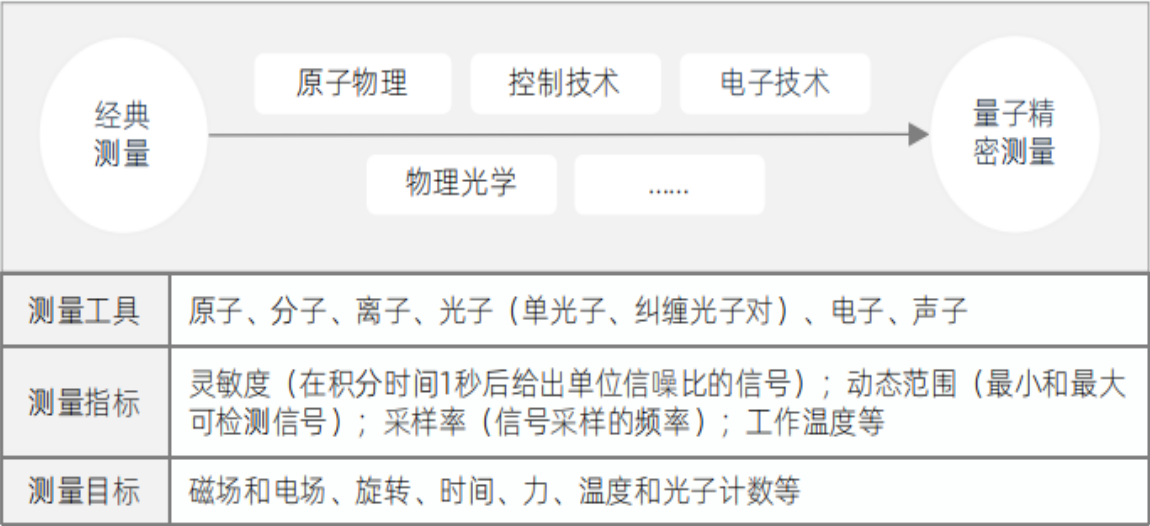
量子精密测量的技术原理
