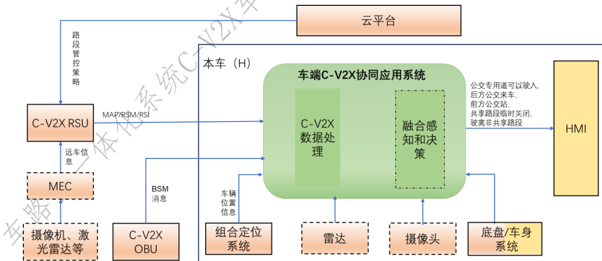
图4-19 公交车道共享场景的功能模块图
