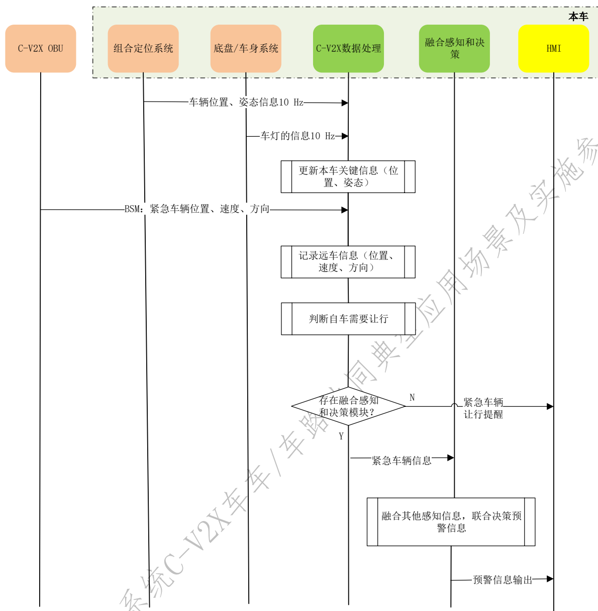
图4-23 紧急车辆优先通行场景的系统间信息流程图
