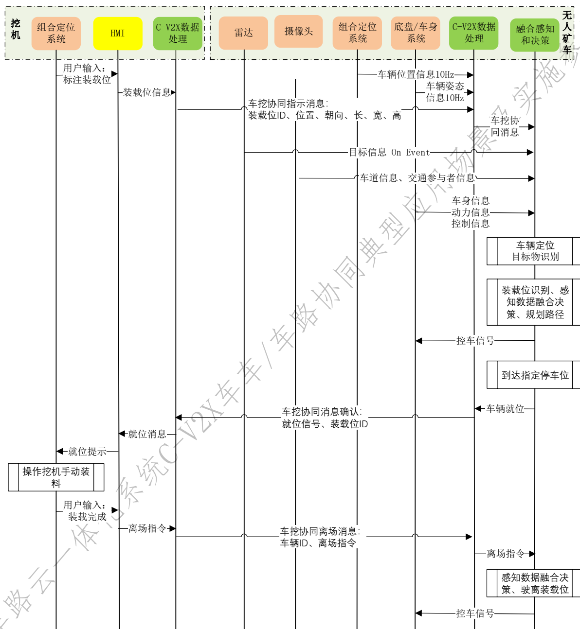
图4-41 矿区车挖协同装载作业场景的系统间信息流图
