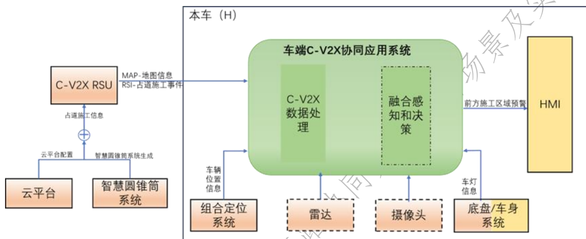
图4-16 圆锥筒信息推送场景的功能模块图
