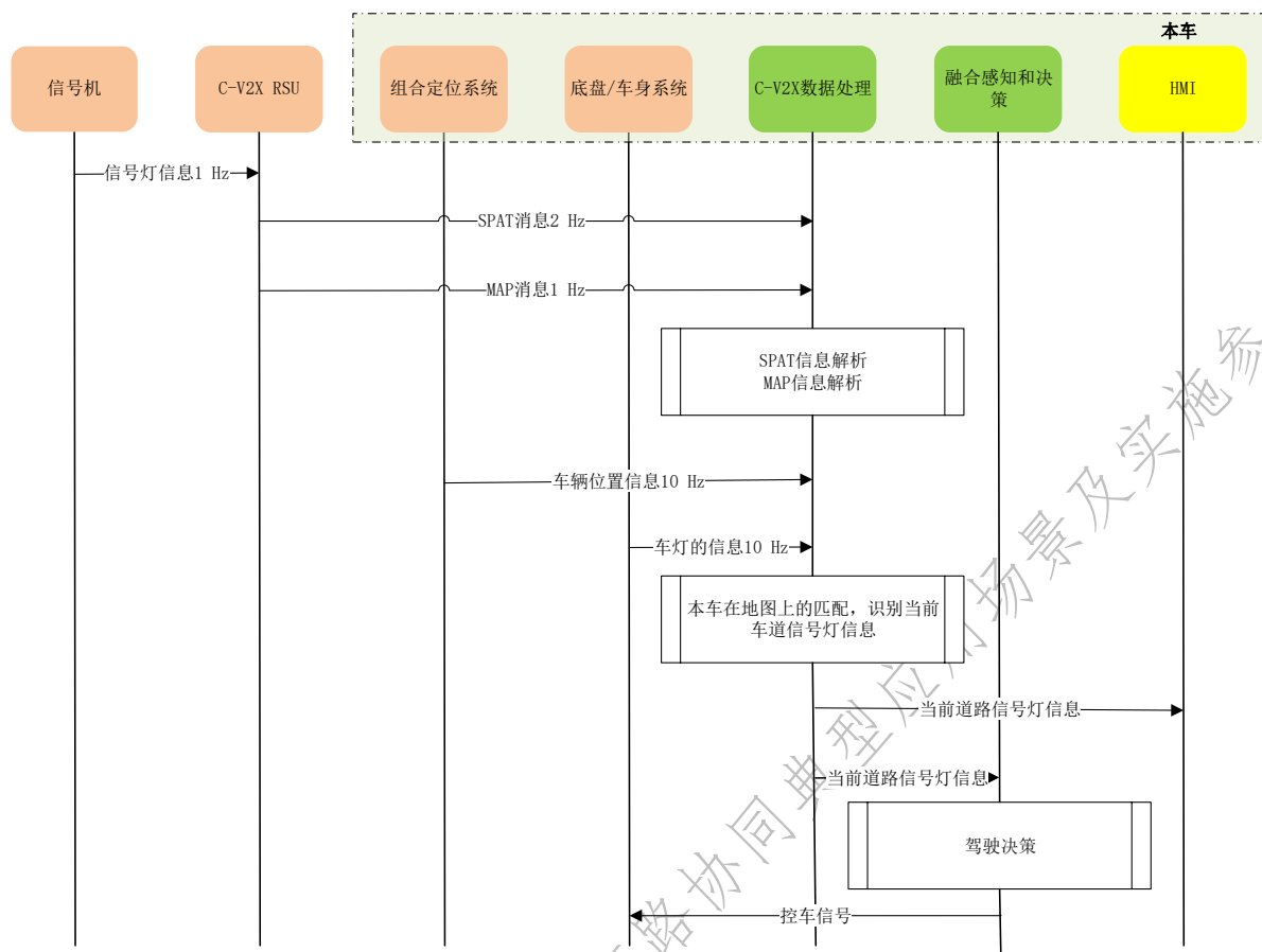
图4-2 交通信号灯上车场景的系统间信息流程图
