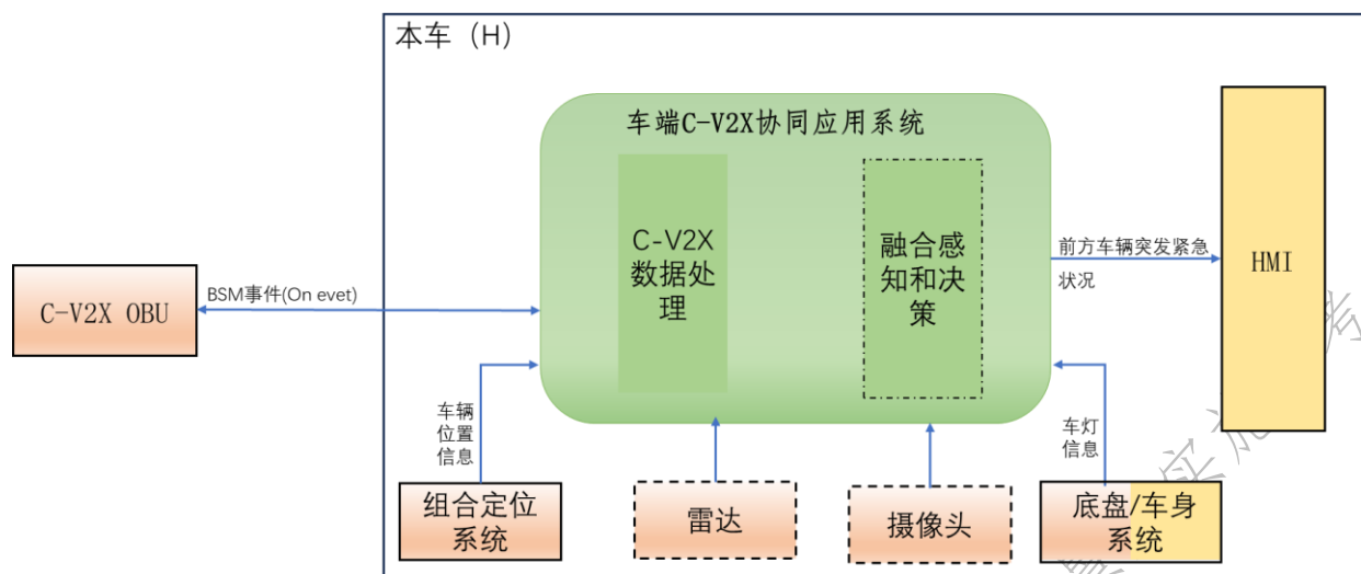
图4-25 前方车辆突发紧急状况场景的功能模块图
