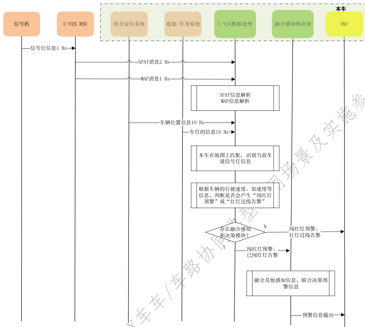
图4-5 闯红灯预警场景的系统间信息流程图
