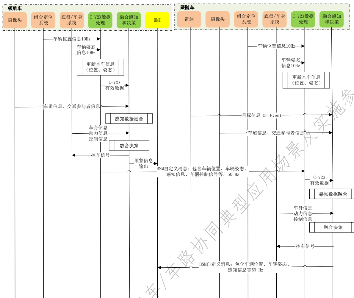
图4-35 车辆智能编队行驶场景的系统间信息流图
