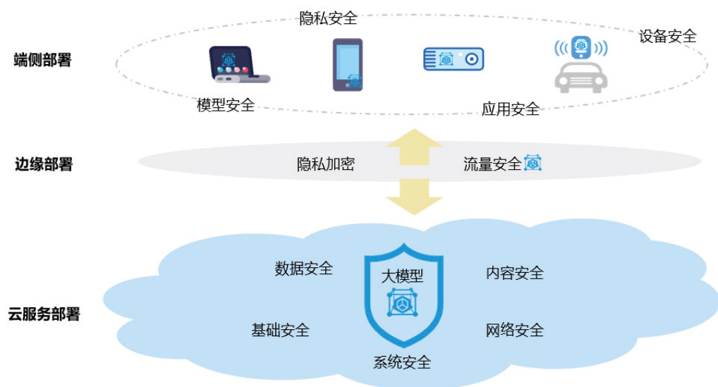
图 2-2 云边端安全架构图
