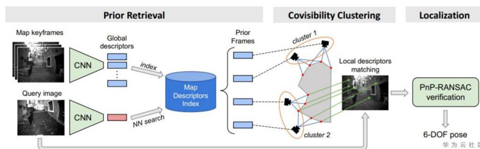
图12 3D 视觉定位中的分级定位
