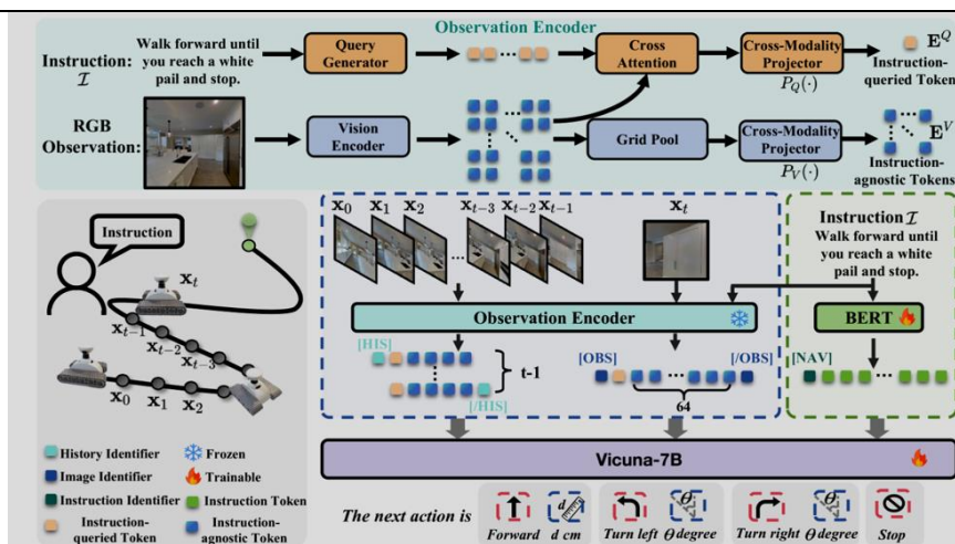
图14 NaVid 架构图
