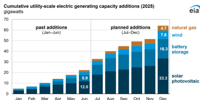
图 10: 2025 年美国新增装机预期
