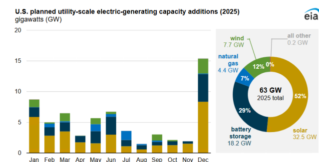
图 8: 2025 年美国新增装机预期
