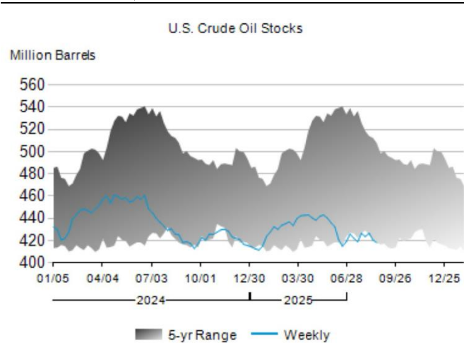
图 33: 美国原油库存 (百万桶)
