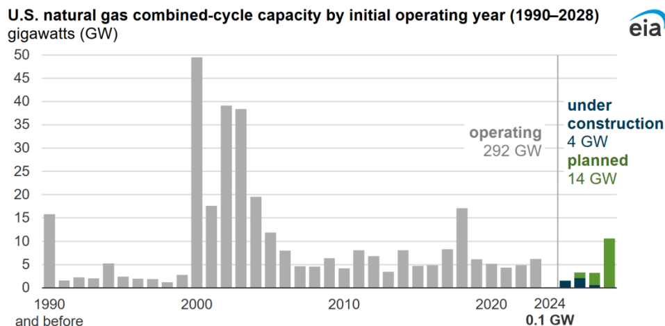
图 6: 美国历年联合循环燃气轮机新装机量
