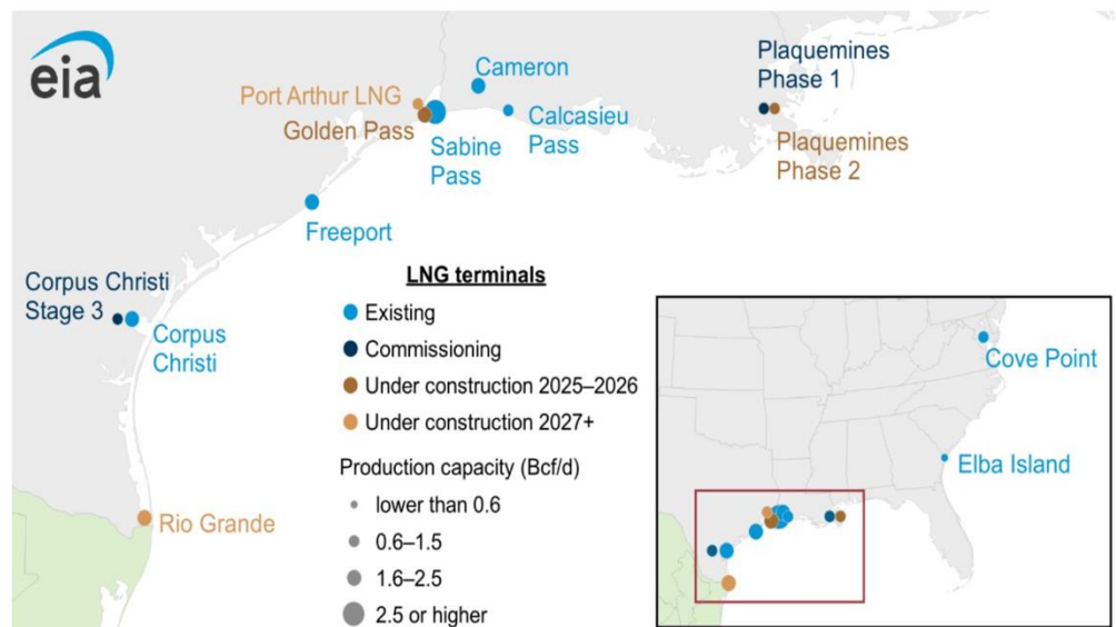
图: 美国液化天然气出口设施情况
