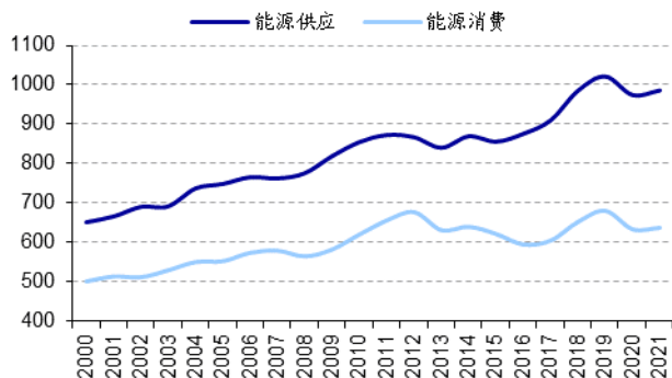
图21 印尼国内能源供应及最终消费（万兆焦耳，2000-2021）
