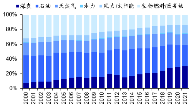
图23 印尼能源供应来源（2000-2021）
