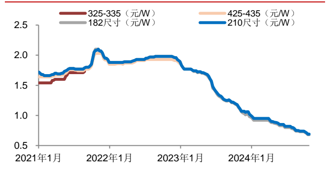
图36: 10月30日182尺寸组件价格0.68元/W, 环比上周持平
