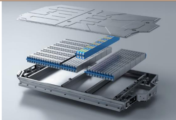
图 32：理想-宁德时代麒麟 5C 电池
