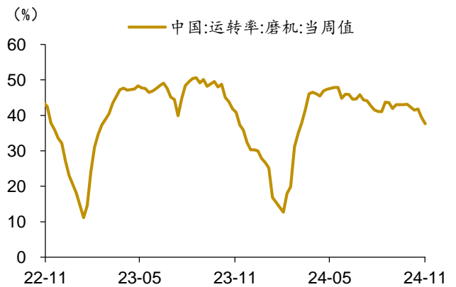
图 18：磨机运转率, %
