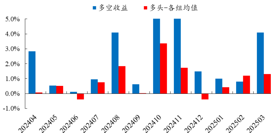
图5：聪明钱因子的“多-空”和“多头-各组均值”月度收益（2024.4-2025.3，多空对冲月度胜率 100.0%）
