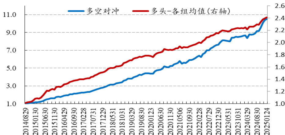
图10：交易行为合成因子的“多-空”和“多头-各组均值”净值稳健（2014.8-2025.3，全市场，行业市值中性）
