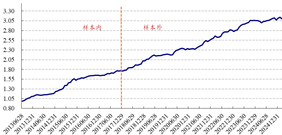
图6：APM 因子的多空对冲净值稳健（2013.6-2025.3，全市场，行业市值中性）
