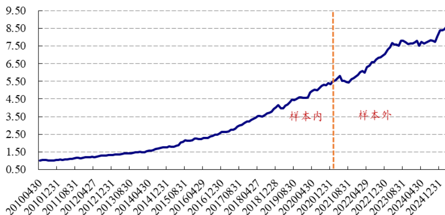
图2：理想反转因子的多空对冲净值稳健（2010.4-2025.3，全市场，行业市值中性）
