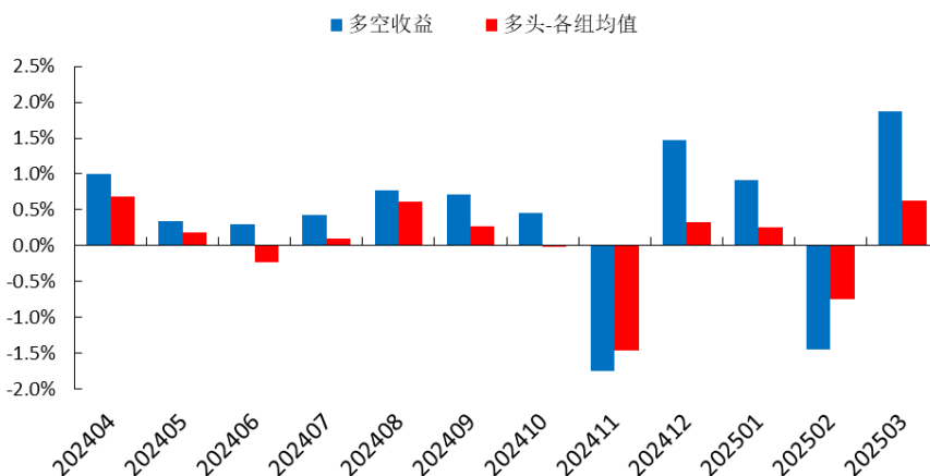
图7：APM 因子的“多-空”和“多头-各组均值”月度收益（2024.4-2025.3，多空对冲月度胜率 83.3%）
