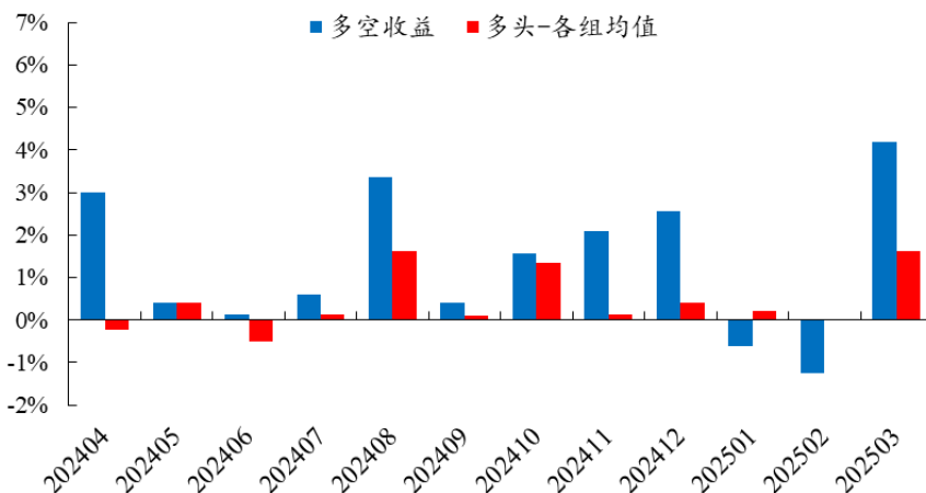
图9：理想振幅因子的“多-空”和“多头-各组均值”月度收益（2024.4-2025.3，多空对冲月度胜率 83.3%）
