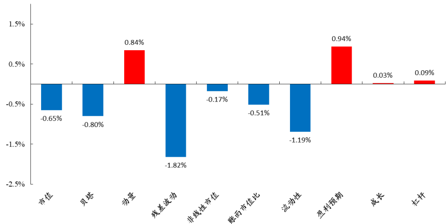
图1: Barra 风格因子收益 (2025 年 3 月)
