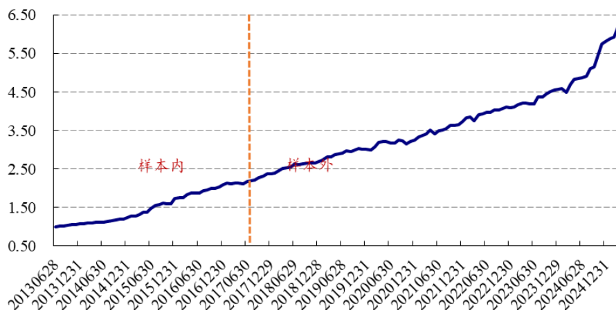
图4：聪明钱因子的多空对冲净值稳健（2013.6-2025.3，全市场，行业市值中性）
