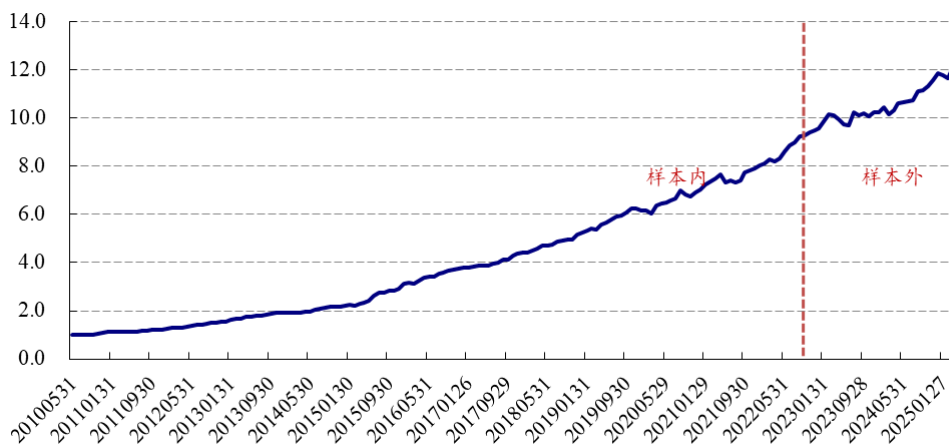
图8：理想振幅因子的多空对冲净值稳健（2010.5-2025.3，全市场，行业市值中性）
