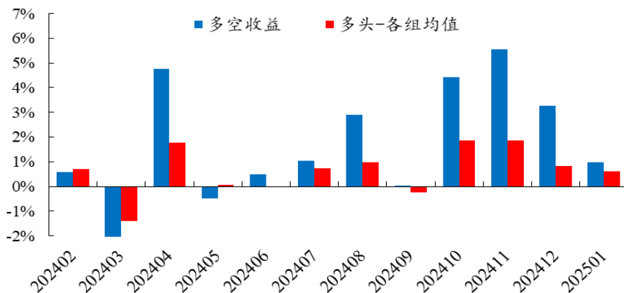
图11：交易行为合成因子的“多-空”和“多头-各组均值”月度收益（2024.4-2025.3，多空对冲月度胜率 83.3%）
