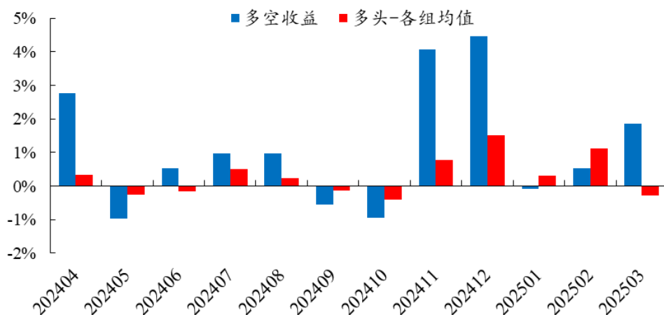
图3：理想反转因子的“多-空”和“多头-各组均值”月度收益（2024.4-2025.3，多空对冲月度胜率 66.7%）
