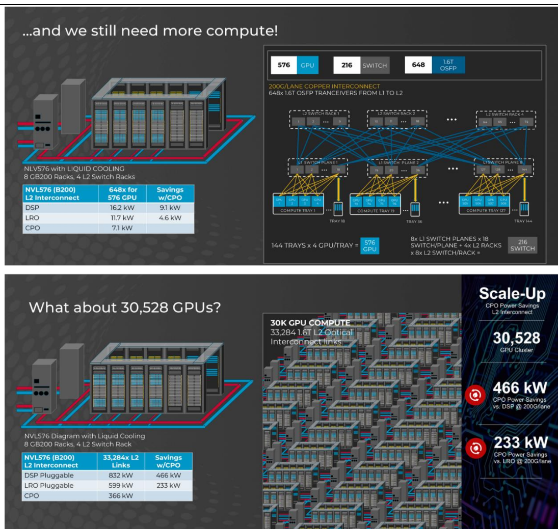
图83：CPO 方案有望有效降低 AI 集群功耗
