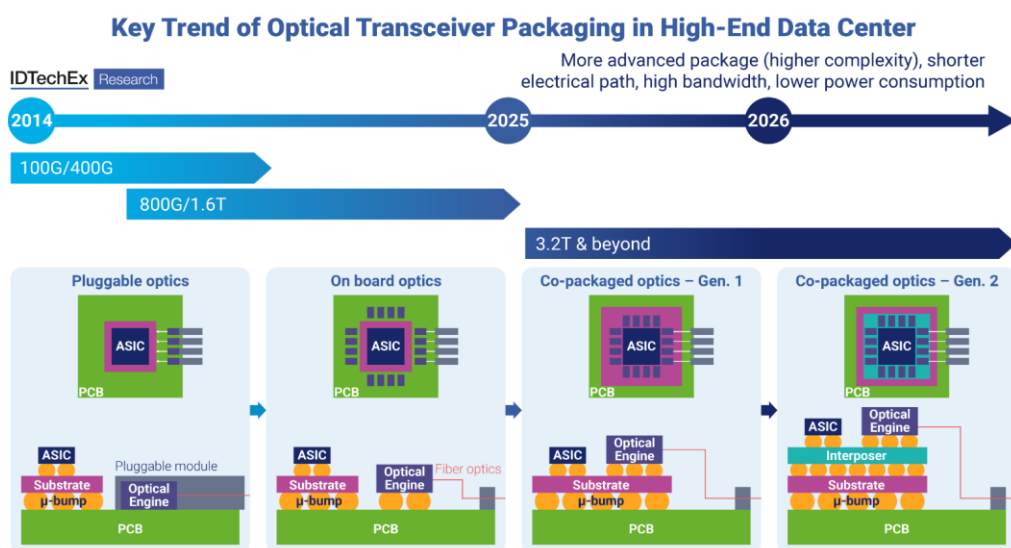
图1：CPO 有望成为未来数据中心互连的重要解决方案
