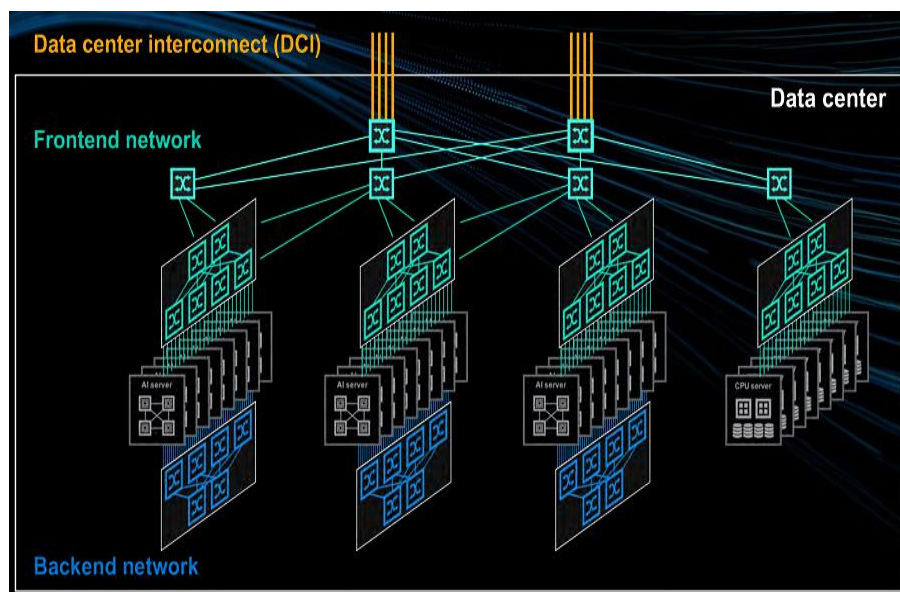
图78：前后端网络组网均带来大量交换机需求
