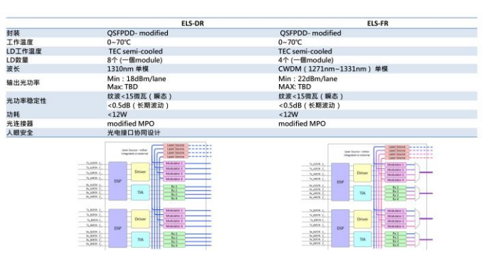
图26： ELS-DR/FR 应用实际由光引擎决定
