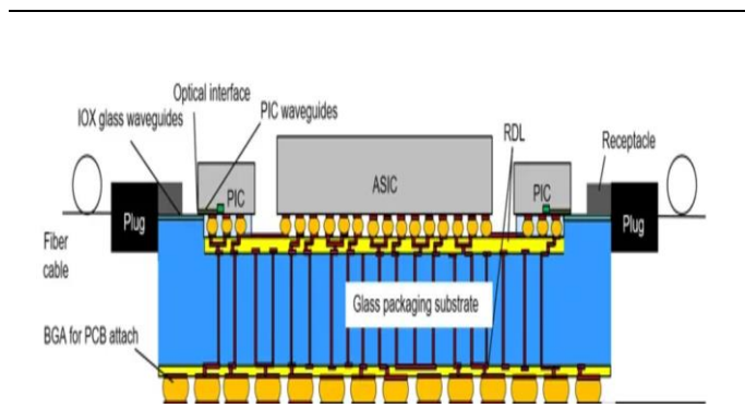
图18：Corning 积极推进玻璃 Interposer
