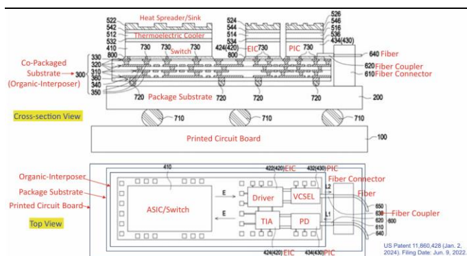
图15: 有机封装利用有机基板作为基材
