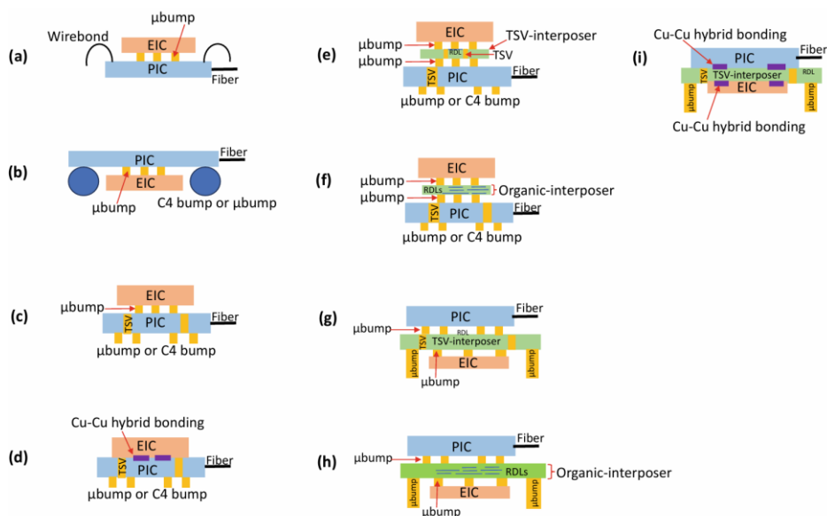
图19：光电芯片通过 3D 封装进行垂直互连
