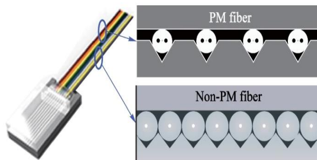
图37：用于光输入的 PM 光纤和用于光输出的非 PM 光纤的混合封装
