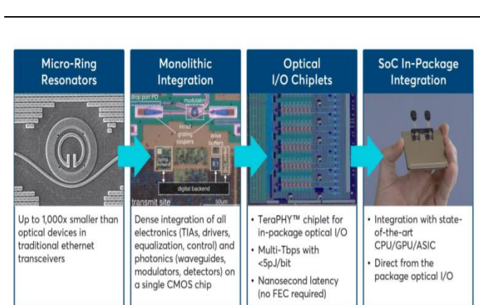
图74: TeraPHY 采用硅光微环调制器
