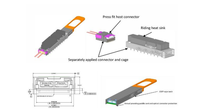
图25： OIF 发布 ELSFP 标准
