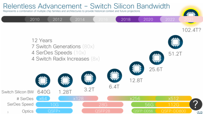
图76：ASIC 带宽约每两年翻一番
