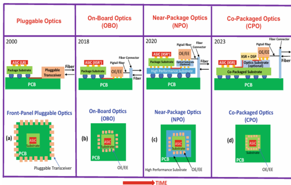
图3：CPO 有望替代传统可插拔光模块
