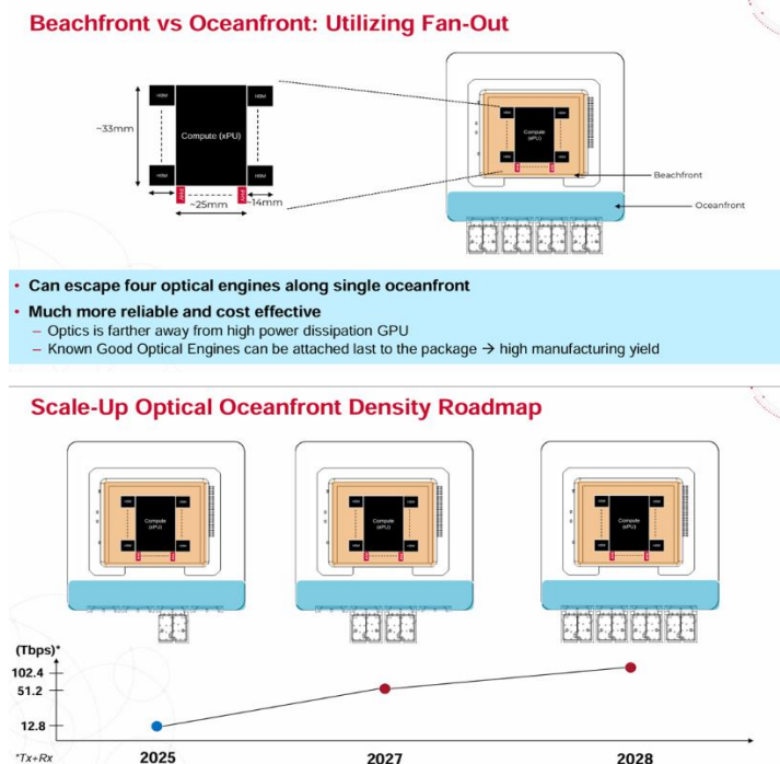
图59: Broadcom 将 CPO 技术进一步拓展到算力芯片
