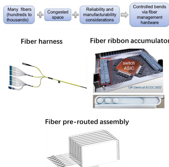
图35：通过部分硬件设计提高光纤可靠性
