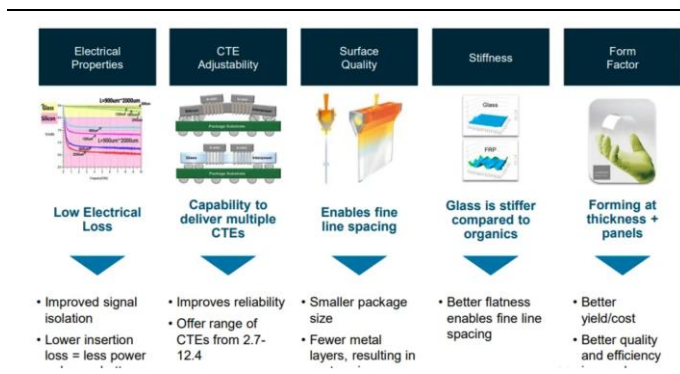
图17：玻璃材料是 Interposer 的优质候选材料
