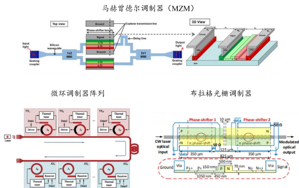
图9：硅光调制器常见构型：MZM、微环调制器、布拉格光栅调制器
