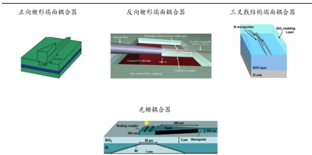
图10：硅光耦合器通常使用端面耦合以及光栅耦合两种方式
