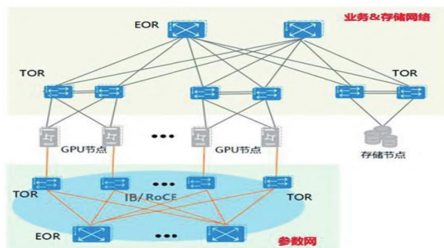
图79: AI 网络架构带动 GPU 互联需求
