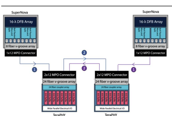
图73: TeraPHY 和 SuperNova 典型链路
