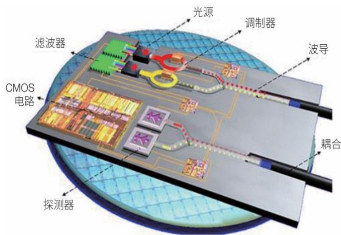
图8：硅光子集成芯片基于硅材料的 CMOS 微电子工艺实现光子器件的集成制备
