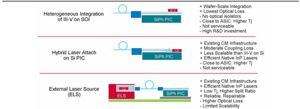
图21：硅光 CPO 主要采用 ELS
