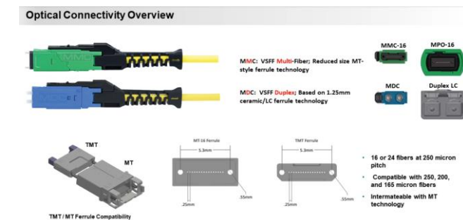
图39：基于 MT 插芯的光纤连接器或成高容量配线需求的重要解决方案
