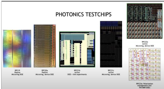
图72: Nvidia 已制造 CPO 各类型测试芯片
