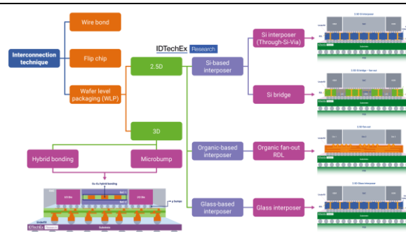
图12: CPO 技术将增加先进封装工艺需求
