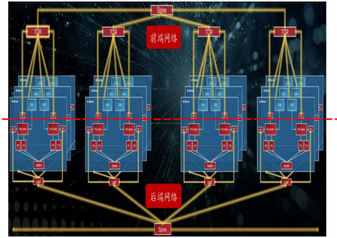
图33: AI 集群组网可分为前端 (Front End) 和后端网络 (Back End)
