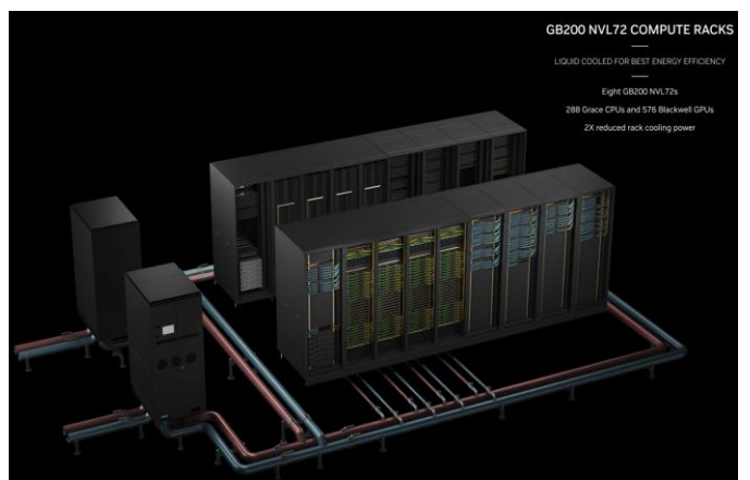
图26：英伟达 NVL576 采用冷板式液冷方案
