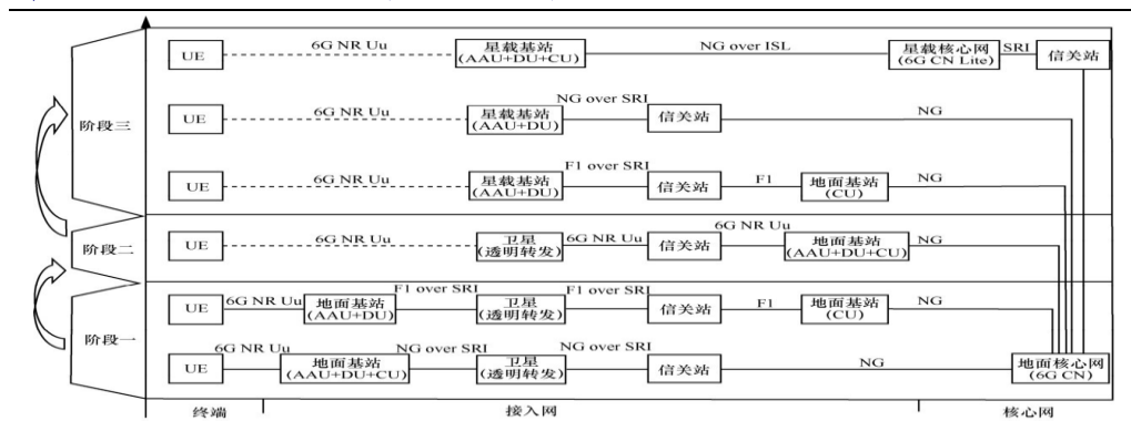
图50：6G 卫星通信网络三阶段演进路线
