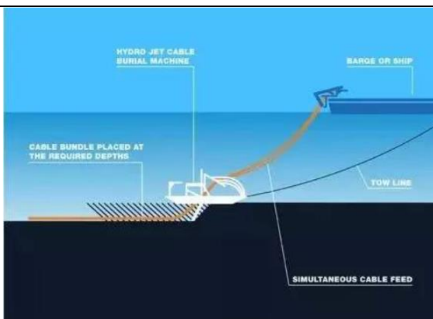
图57：缆敷设主要包括电缆路由勘查清理、海缆敷设和冲埋保护三个阶段
