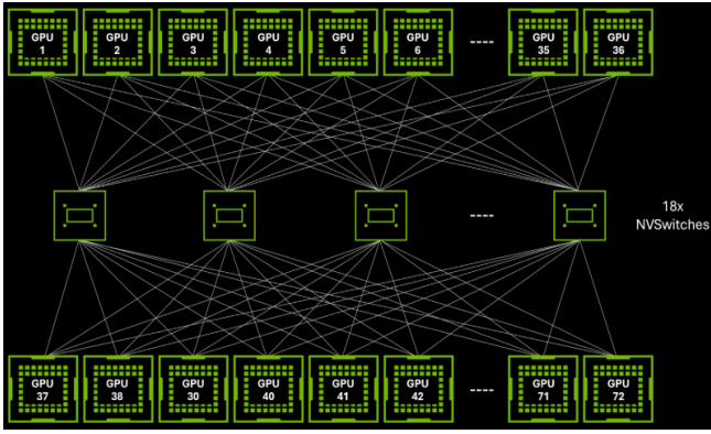
图39：18个 NVSwitches 连接 72 个 GPU
