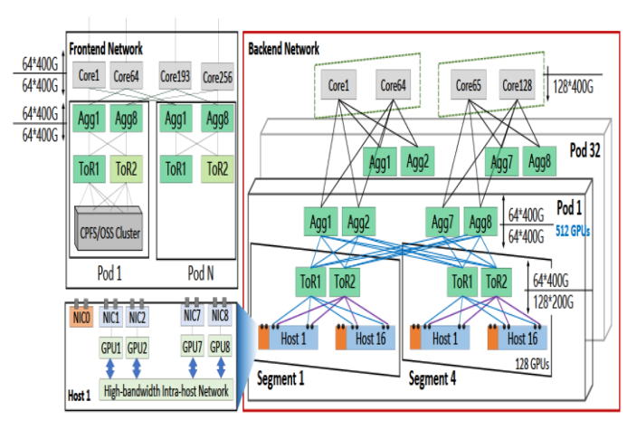
图34: 前后端网络组网均带来大量交换机需求
