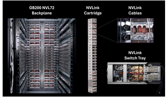
图40：NVL72 背部通过 5000 多根铜缆互联
