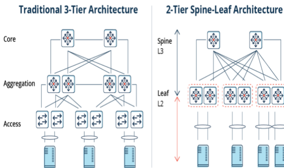
图15: 传统三层网络架构向 Spine-Leaf 架构转变
