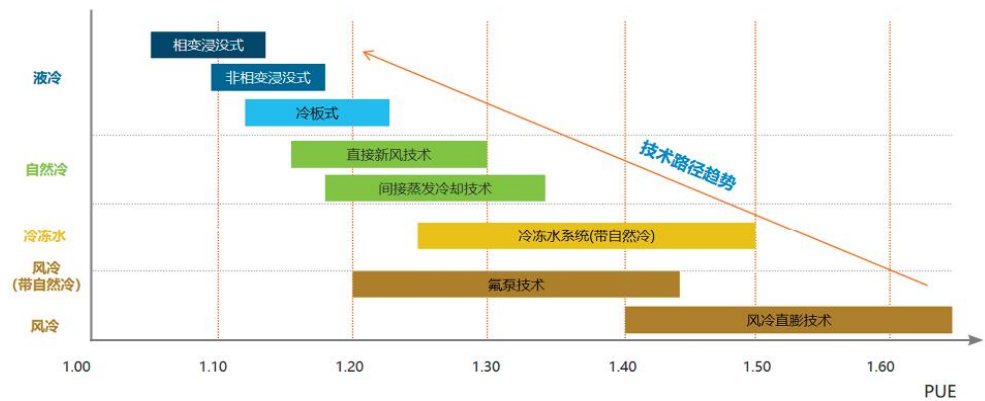
图23：数据中心制冷技术逐渐向液冷发展
