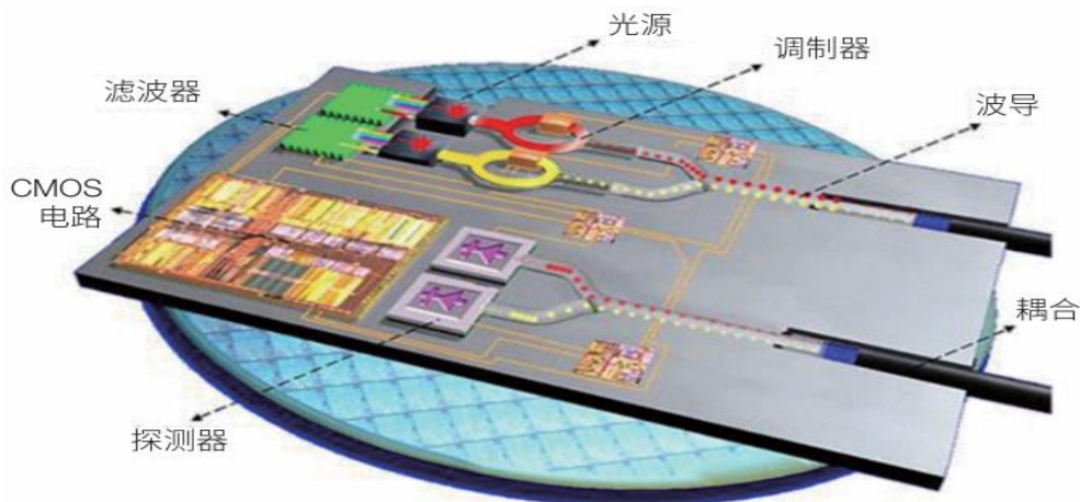
图19：硅光子集成芯片基于硅材料的 CMOS 微电子工艺实现光子器件的集成制备
