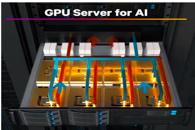
图25：GPU (AI) 服务器采用冷板式液冷散热
