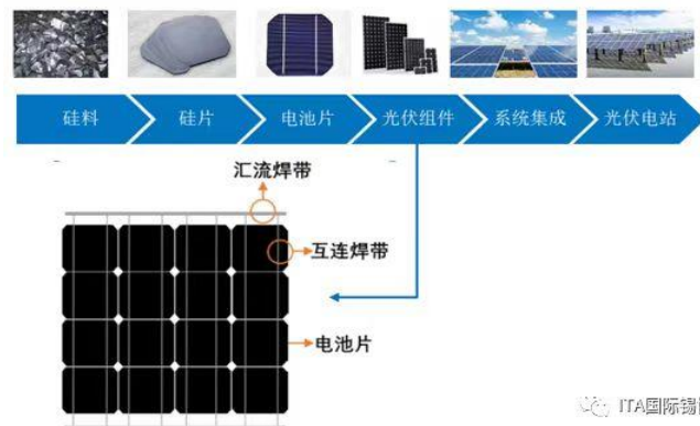
图51: 焊带在光伏电池中的应用
