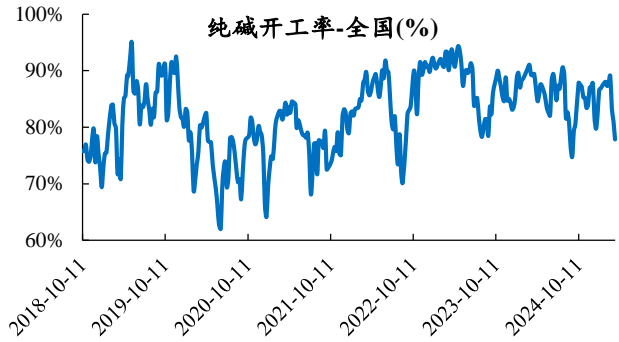
图43: 本周全国纯碱开工率环比下降 3.25pct
