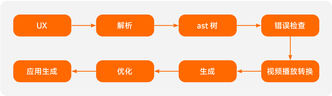
图 4.7-5 编译工具链
