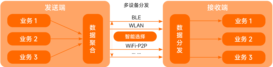
图 3.1-5 多设备分发架构
