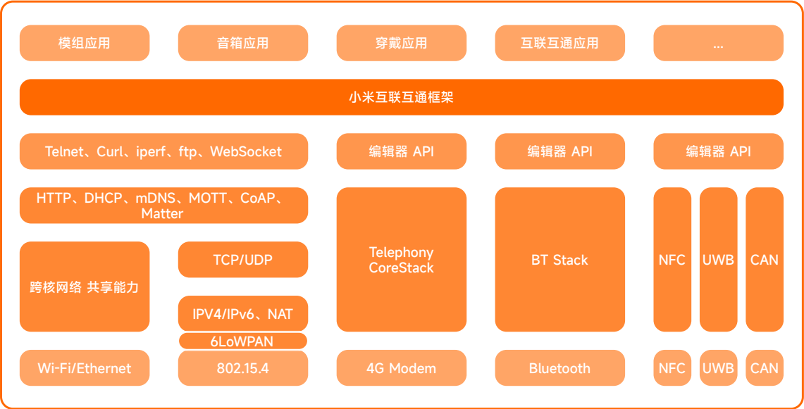
图 5.2-11 Vela 通信子系统
