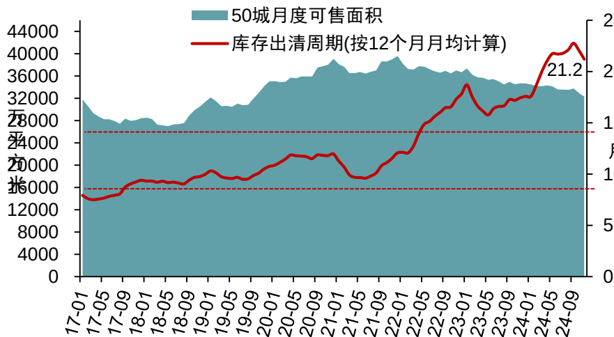
图表10：50个代表城市商品住宅短期库存出清周期走势
