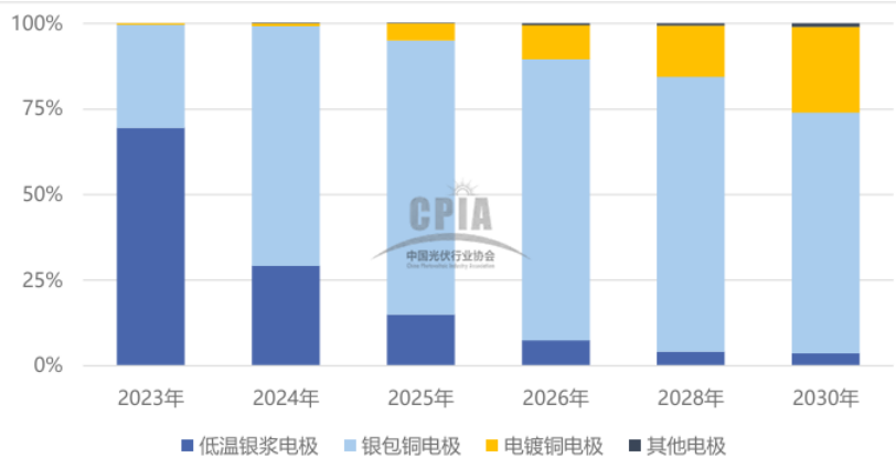
图：HJT电池片金属电极技术市场占比预测
