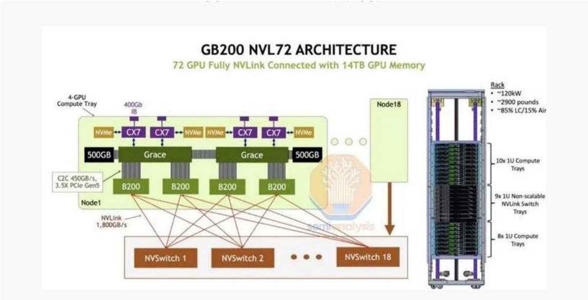
图：NVL72结构
