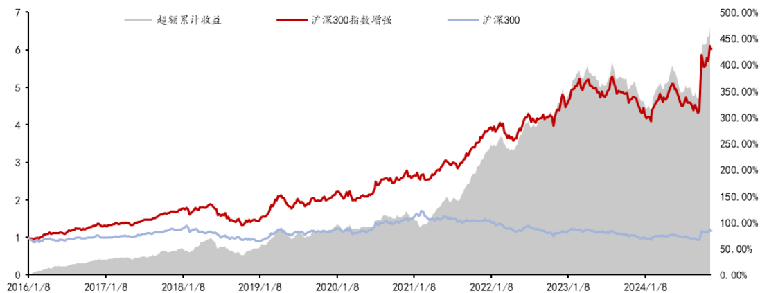
图表35：沪深 300 指数增强绩效跟踪（左轴：沪深 300 指数增强，沪深 300；右轴：超额累计收益率）
