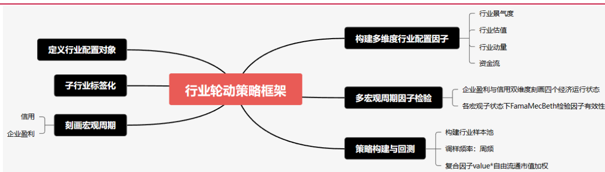
图表30：量化行业轮动策略框架
