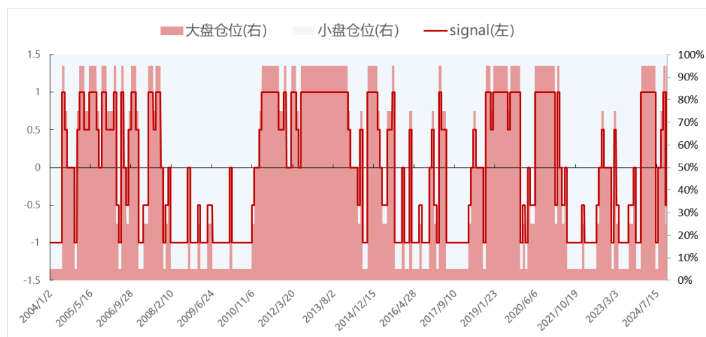
图表17: 信号值与大小盘仓位时序变化
