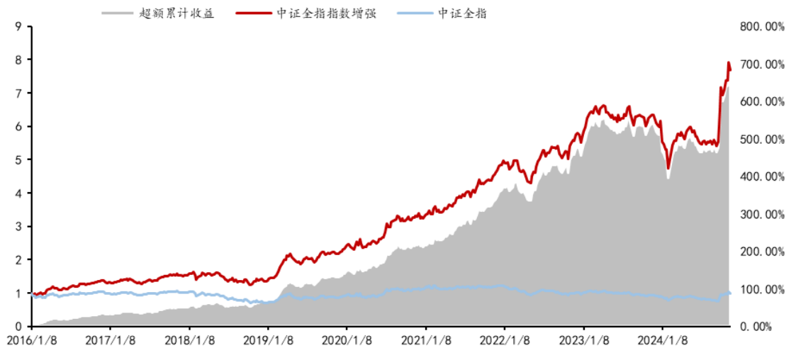
图表41：中证全指指数增强绩效跟踪（左轴：中证全指指数增强，中证全指；右轴：超额累计收益率）
