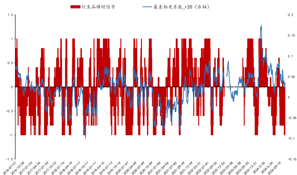
图表12：基于基差的股指期货择时信号
