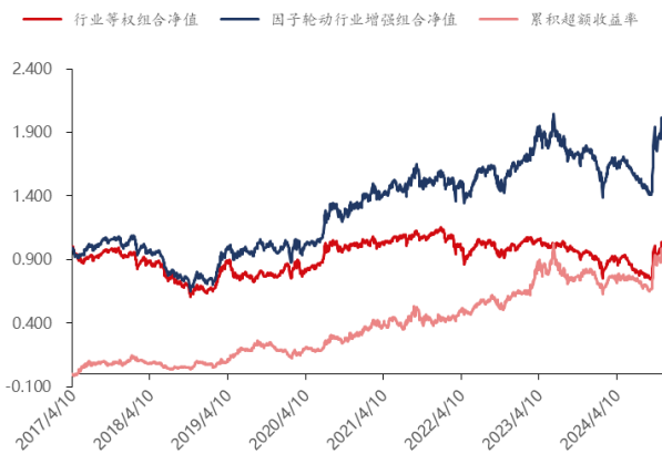
图表26：行业轮动组合月度净值走势(无剔除)
