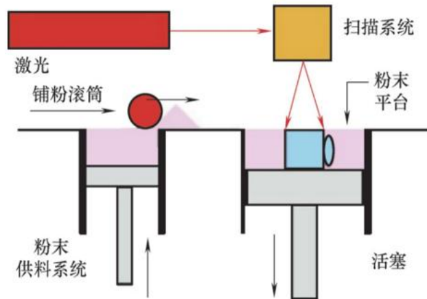
图 4：选区激光烧结（SLS）成形原理图
