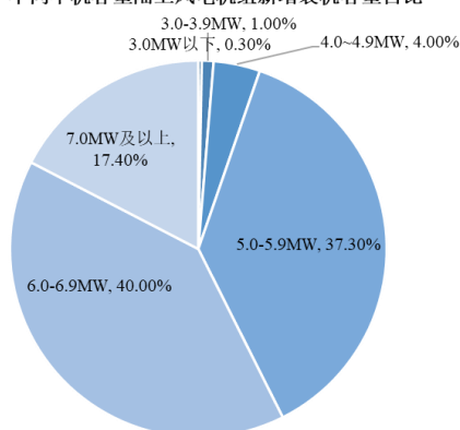
2024年不同单机容量陆上风电机组新增装机容量占比
