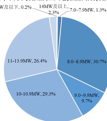
2024年不同单机容量海上风电机组新增装机容量占比
