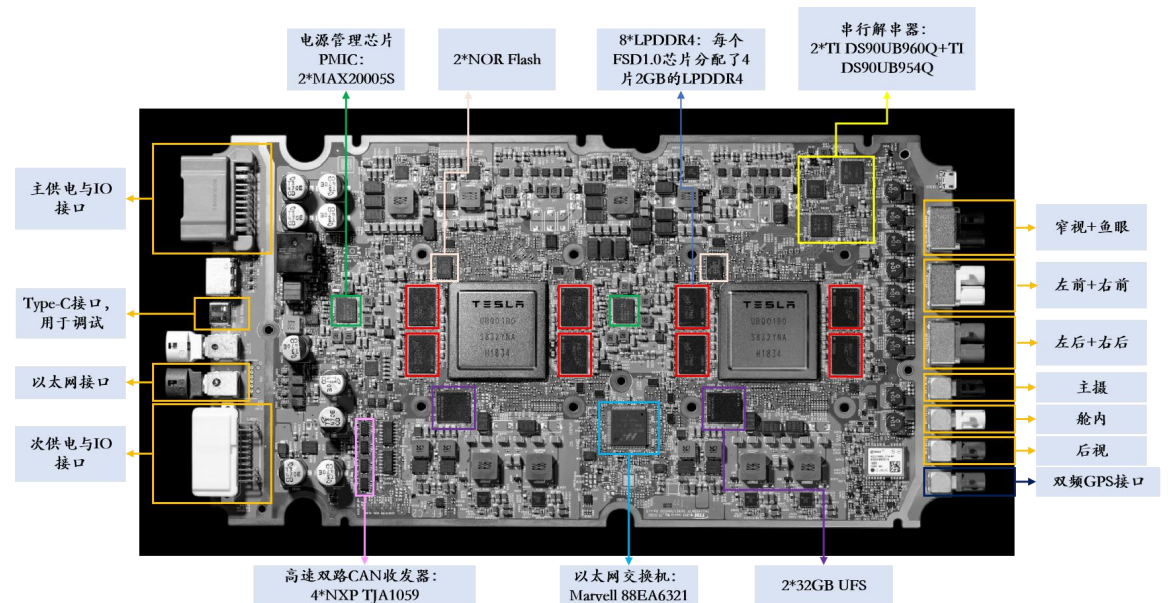
智驾域控包括大量电子元器件：以特斯拉HW3.0为例
