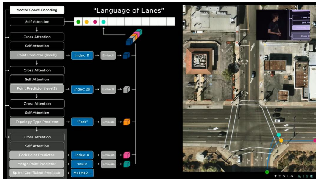
特斯拉Lanes network模型语义模块架构
