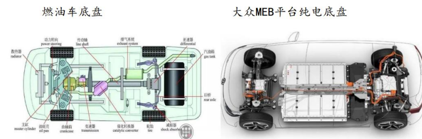
图3：燃油车平台和纯电平台底盘对比
