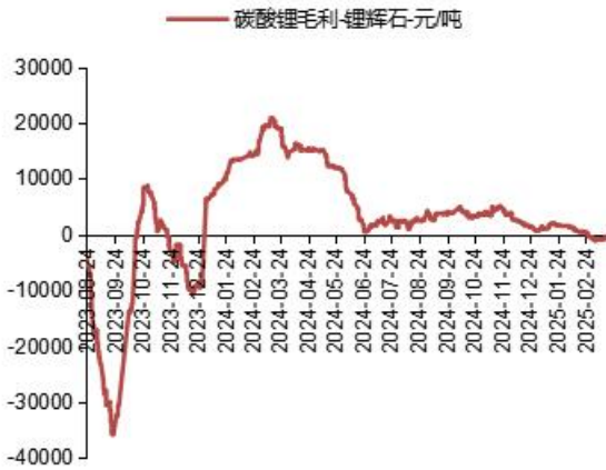
图表 37：以锂辉石为原料的冶炼毛利走势(元/吨)
