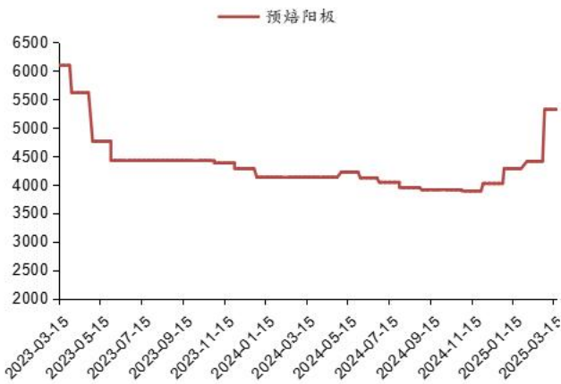
图表 18: 预焙阳极价格走势 (元/吨)
