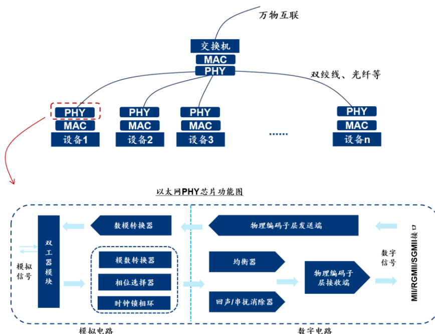
图表40：以太网 PHY 芯片工作原理示意图
