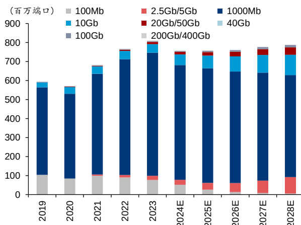
图表34：全球园区企业交换机市场结构（按端口速率）
