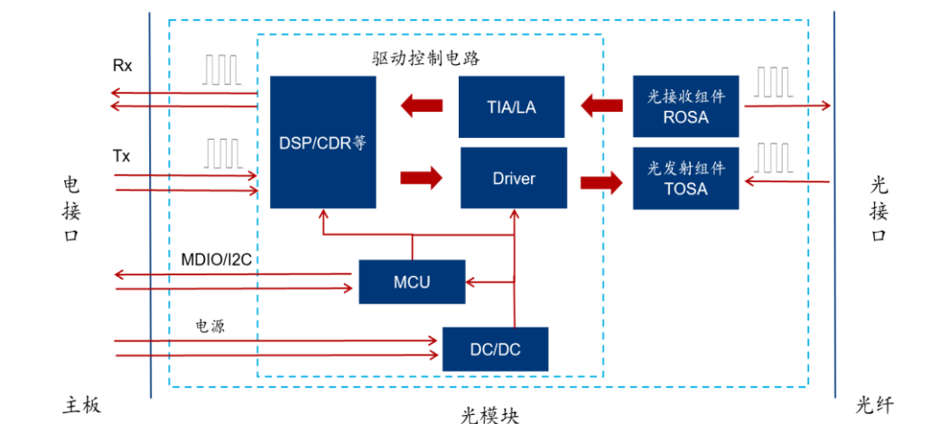
图表12：光模块组成结构示意图
