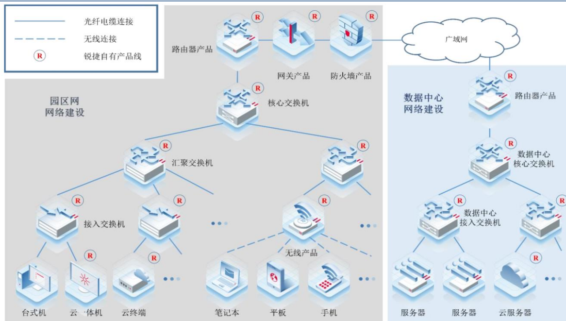
图表28：交换机在园区网络和数据中心网络中的作用
