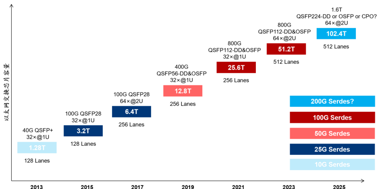
图 30：以太网交换芯片容量
