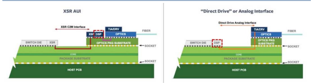
图表20: CPO 架构方案
