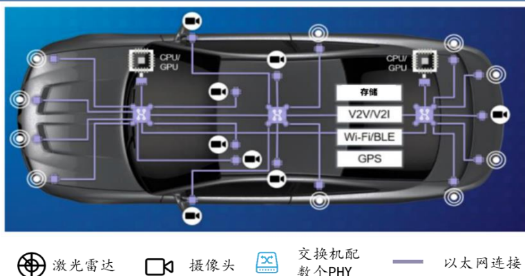
图表44: AQUANTIAADAS 系统以太网架构
