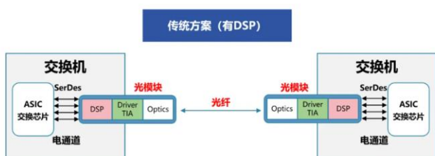
图表18：传统光模块方案结构示意图
