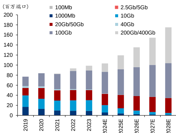
图表33：全球数据中心交换机市场结构（按端口速率）
