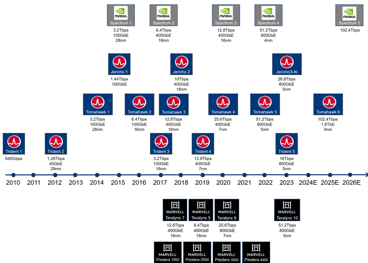
图表38：以太网交换芯片推出时间表
