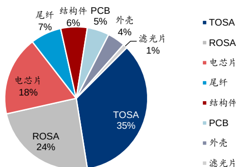
图表17：光模块成本构成
