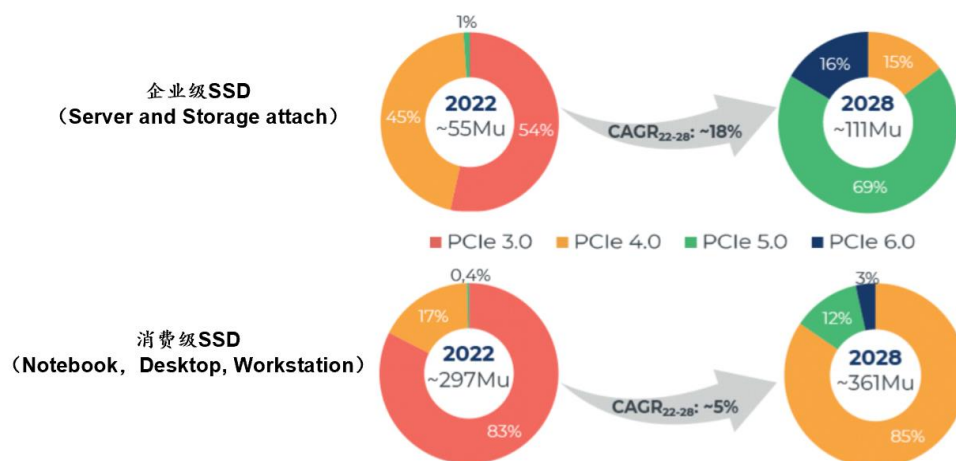
图表66：全球 PCIe 接口企业级 SSD 和消费级 SSD 市场出货量
