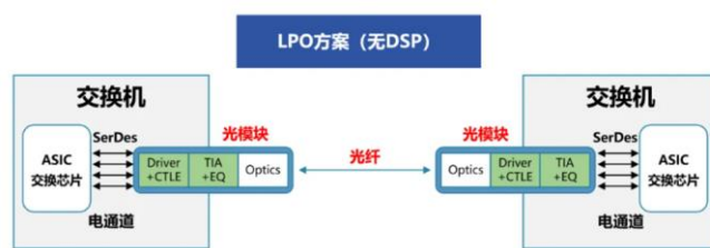
图表19：LPO 光模块方案结构示意图
