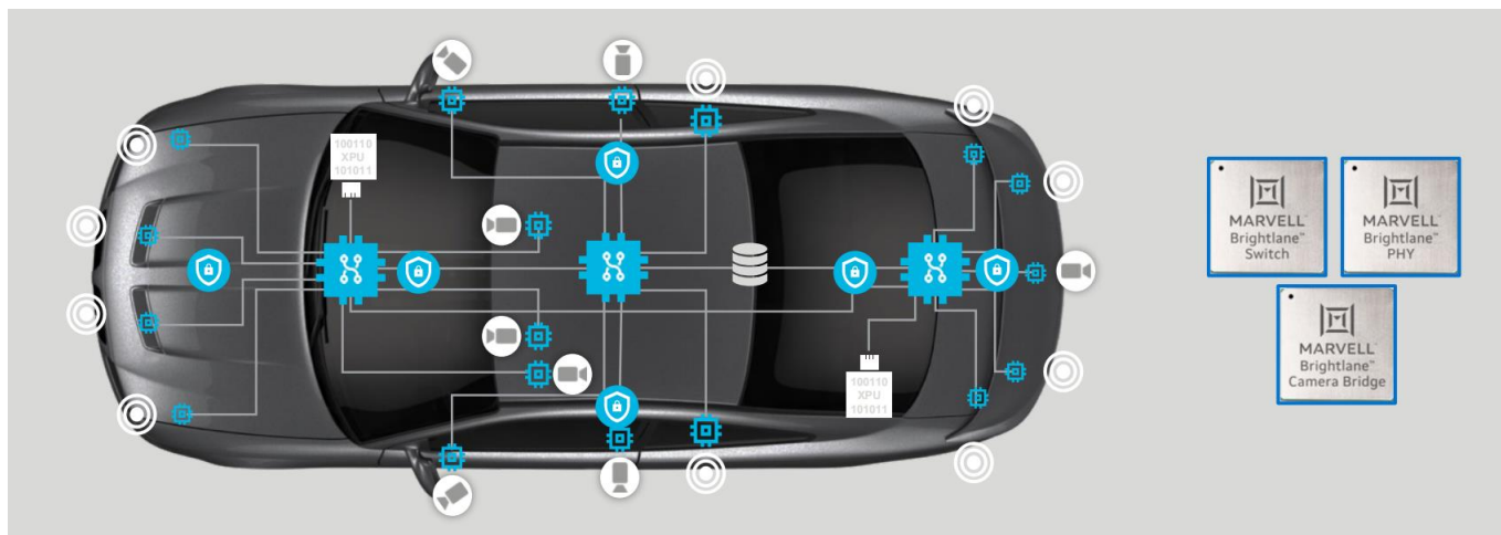
图表39：Marvell 交换芯片在车载以太网应用示意图
