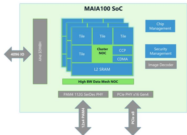
图 17: 微软 Maia 100 芯片架构
