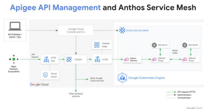
图表93：使用 Apigee API 构建现代应用和架构
