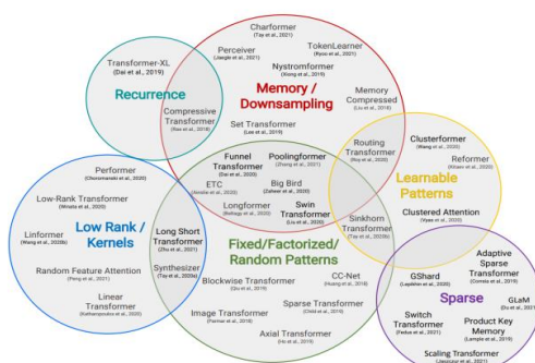
图表49：基于 Transformer 开发的高效模型（按技术和应用分类）
