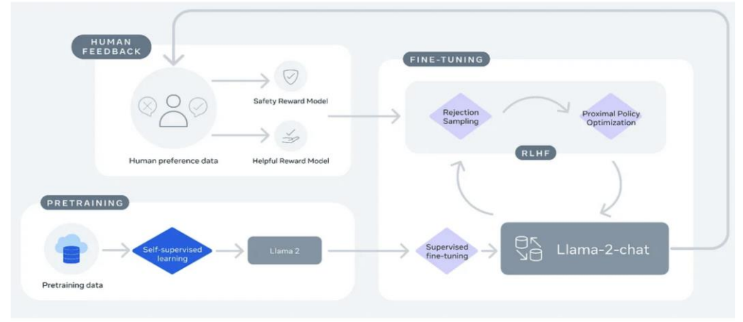
图表33: LLaMA 2 架构图
