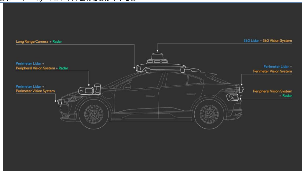
图表114：Waymo 第五代车型传感器分布示意图
