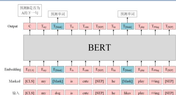
图表50：BERT 模型预训练过程
