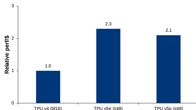
图表14：谷歌历代 TPU 训练大模型每美元相对性能比较
