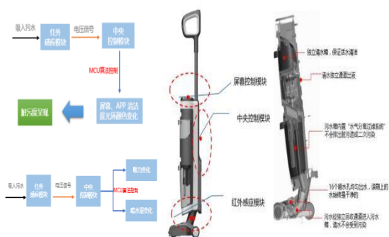
图表22：添可洗地机1.0的结构设计及原理示意图
