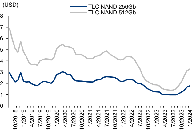
图表90: 主流 TLC NAND 现货价格
