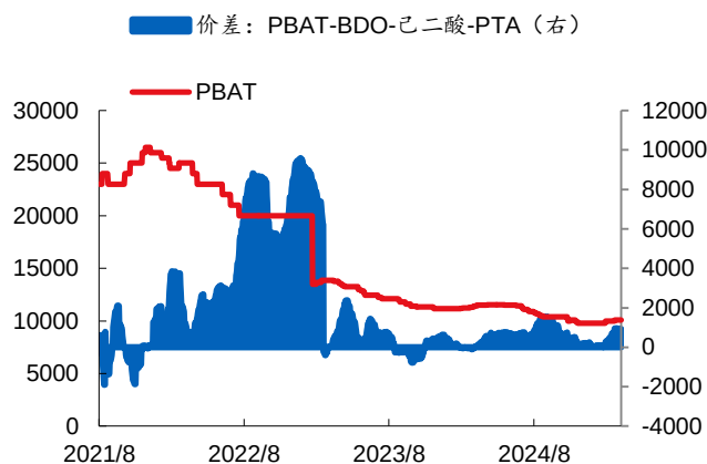
图表 40 PBAT 价格与价差
