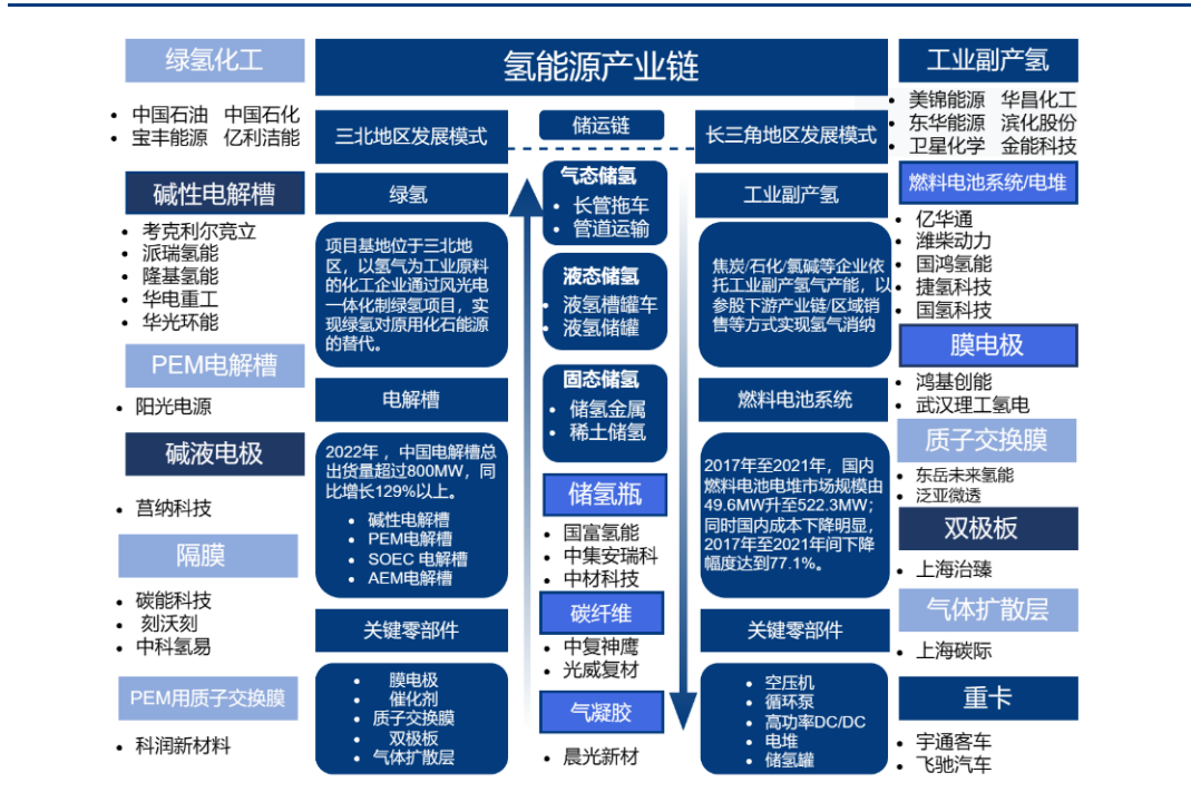
图表 17 氢能行业重点标的一览
