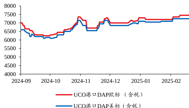
图表 36 UCO 港口价格
