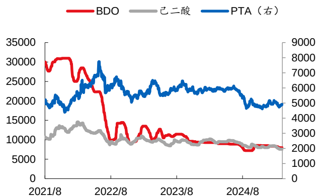
图表 41 PBAT 原料价格
