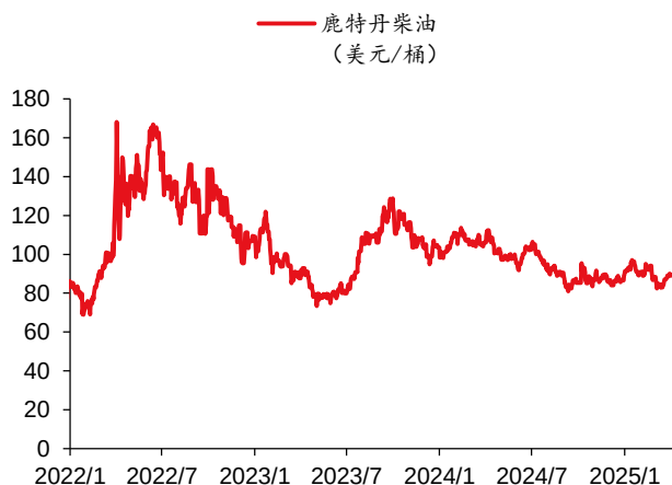
图表 39 鹿特丹柴油价格
