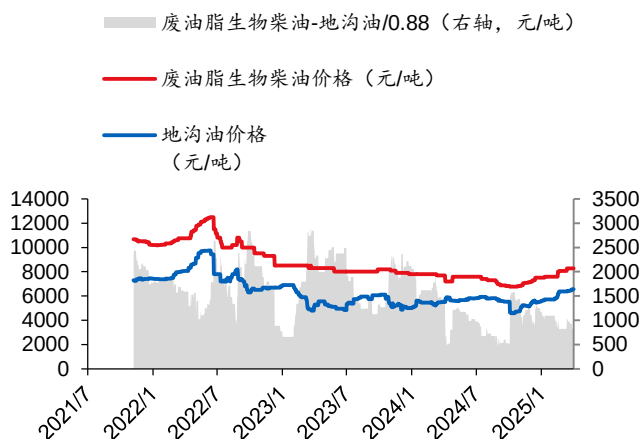
图表 37 废油脂生物柴油价差
