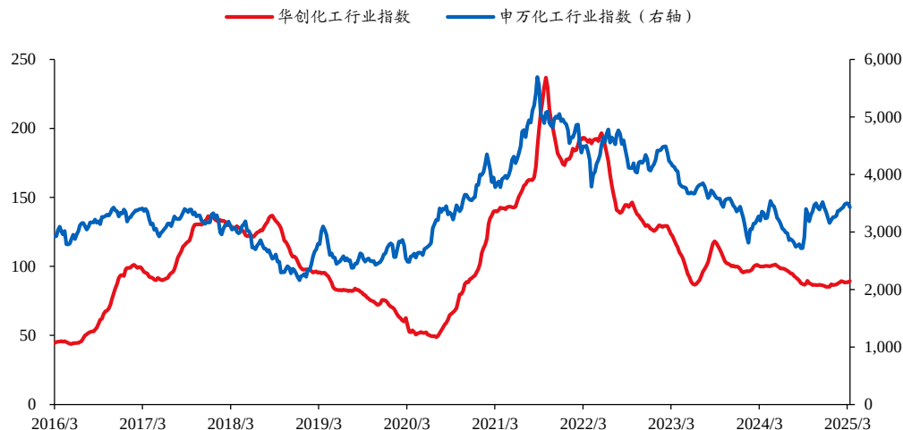
图表 1 本周华创化工行业指数 89.31，环比+0.96%，同比-10.56%
