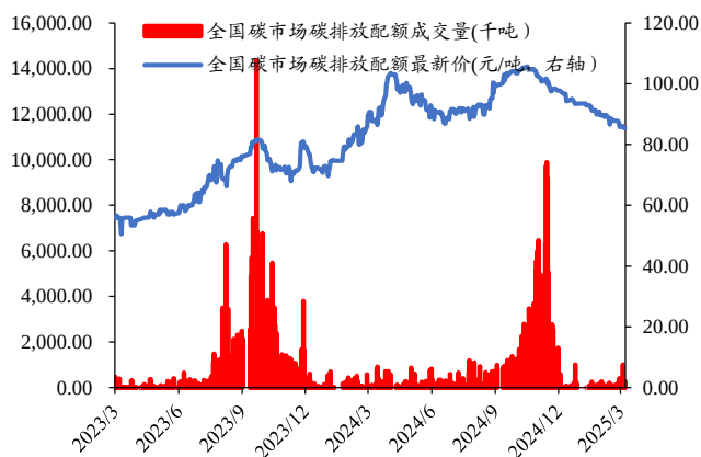
图表 18 本周全国碳市场排放交易价格环比-0.85%
