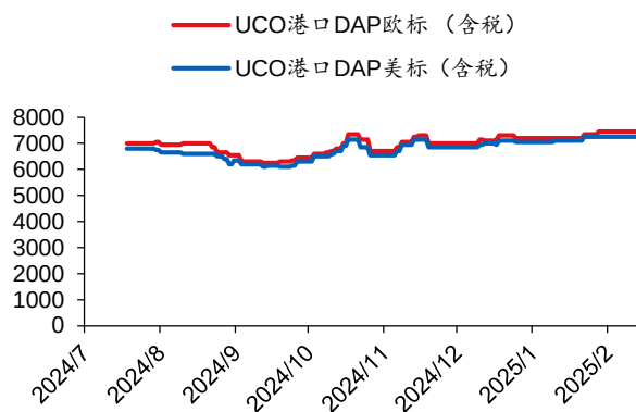
图表 36 UCO 港口价格
