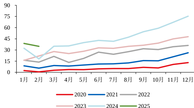
图表 8 2 月国内动力锂电池装机量 34.9GWh（GWh）
