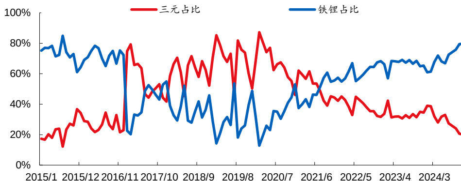
图表11 11月LFP装机占比79.7%
