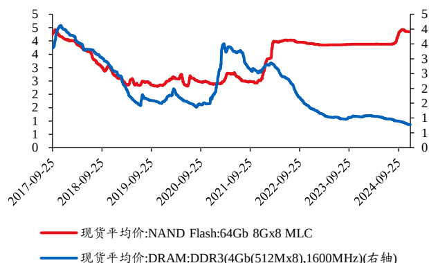
图表 69 本周 DRAM 价格环比持平
