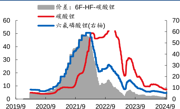
图表 14 本周 6F 价格不变（万元/吨）
