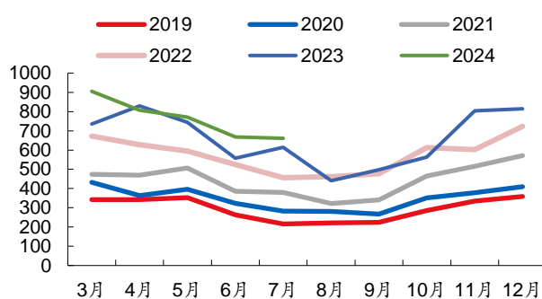
图表 21 7 月风电产量 660.9 亿千瓦时 (亿千瓦时)
