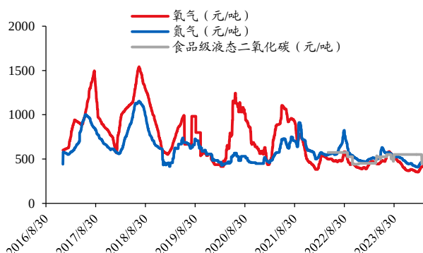
图表 59 本周氧气价格环比上涨，氮气价格环比下跌
