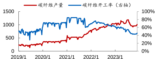
图表 26 本周碳纤维产量上升（吨）
