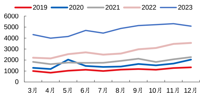
图表 20 12 月光伏电池产量 5083 万千瓦（万千瓦）
