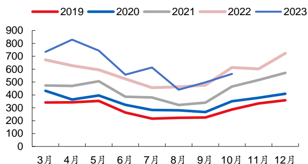
图表 21 9月风电产量563亿千瓦时(亿千瓦时)
