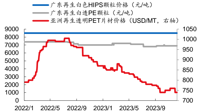
图表 47 再生 PET 价格
