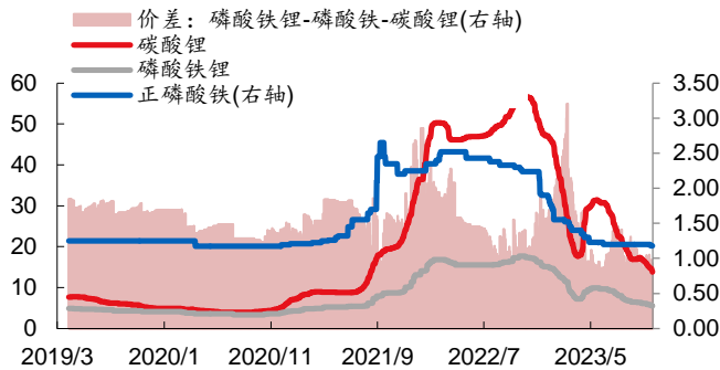
图表 12 本周磷酸铁锂价格下降（万元/吨）
