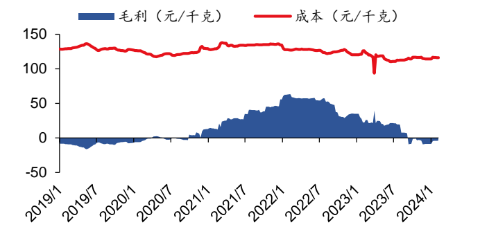
图表 29 本周碳纤维行业毛利降低 (元/千克)
