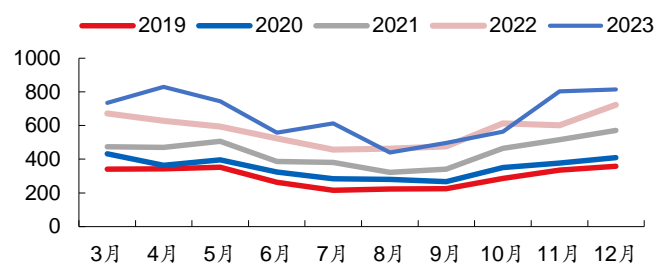
图表 21 12 月风电产量 814 亿千瓦时 (亿千瓦时)
