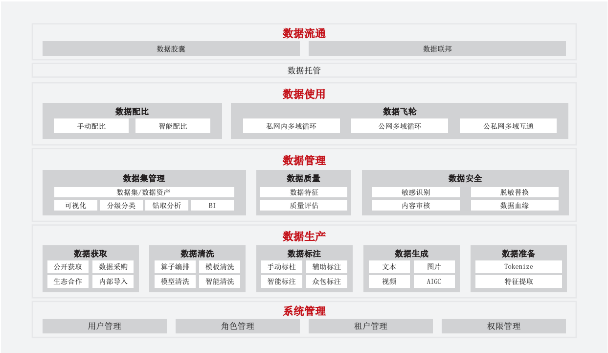
图 5 数据平台
