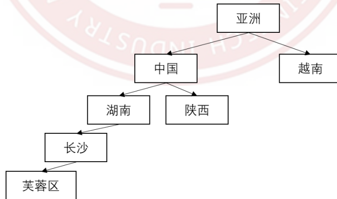
图 7 地区泛化树实例
