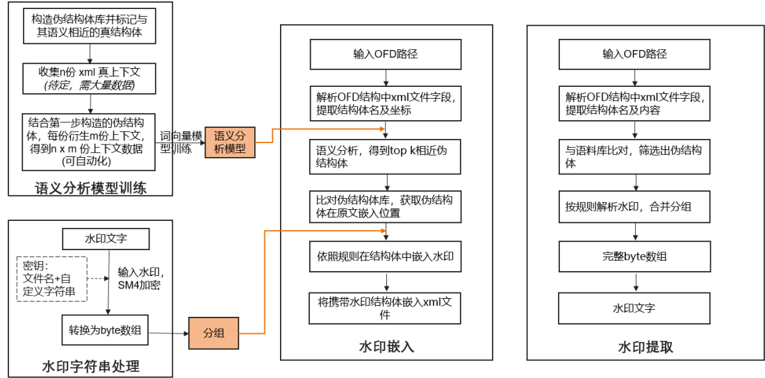
图 11 基于伪结构体的 OFD 隐式水印算法流程
