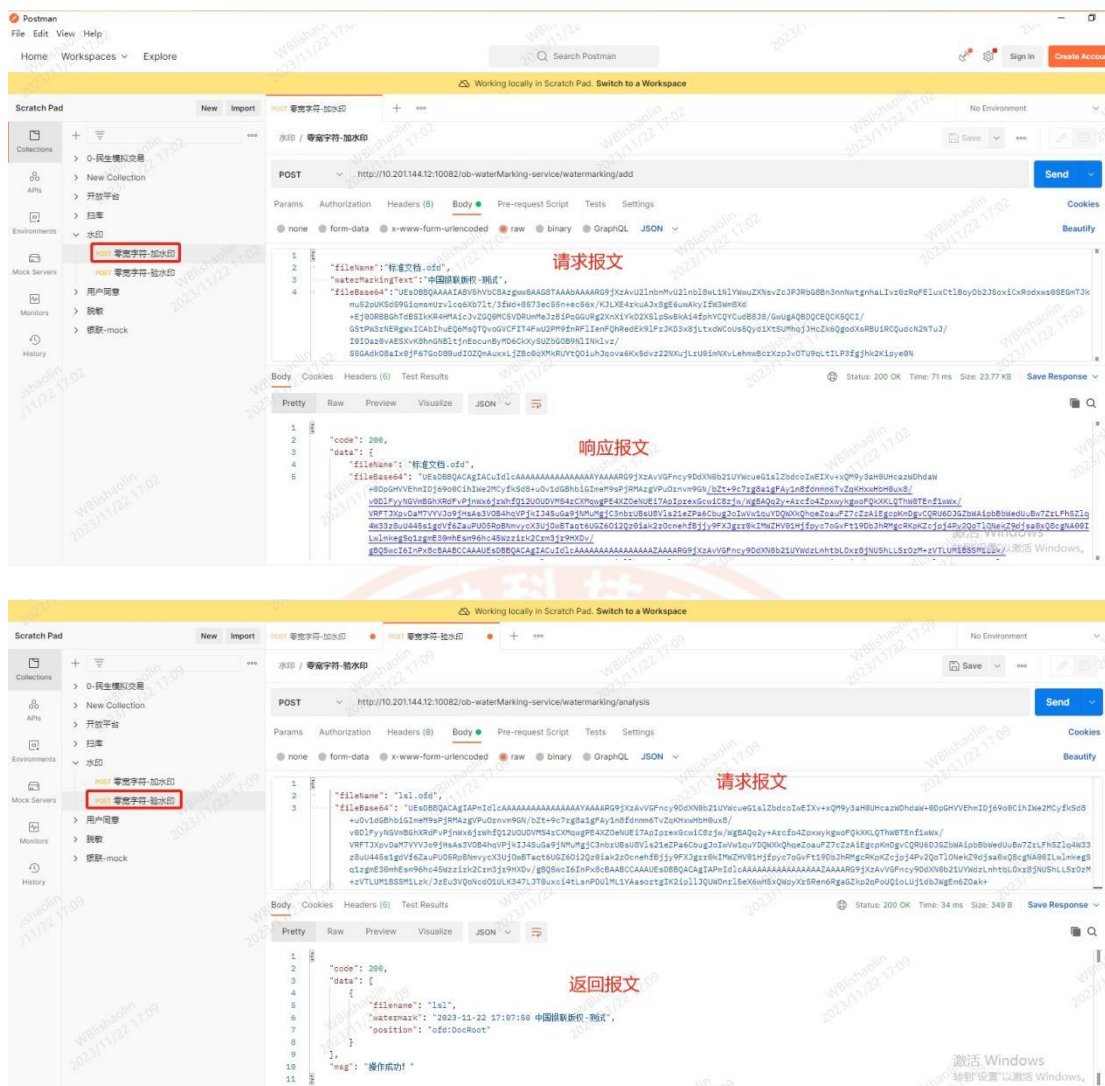
图 13 OFD 水印测试结果
