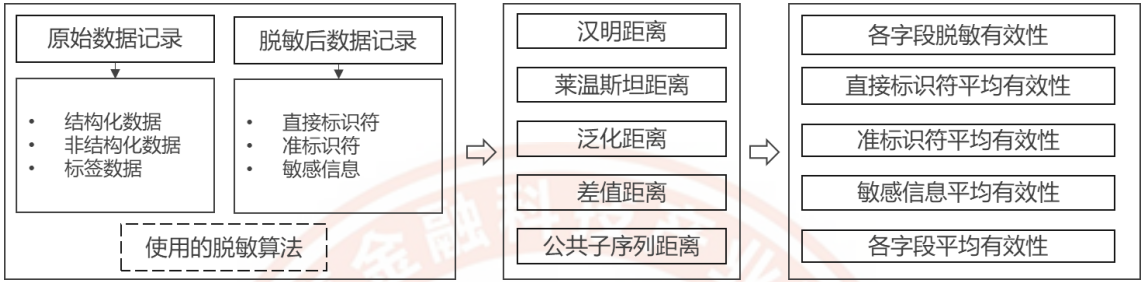
图 6 有效性指标计算流程
