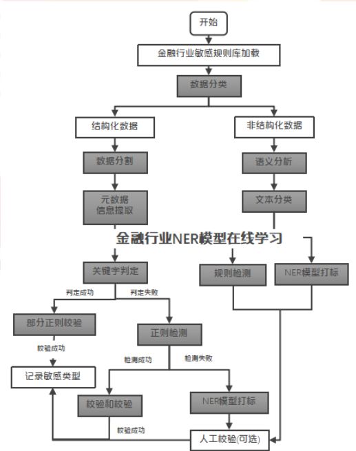
图 3 分类分级规则库处理流程
