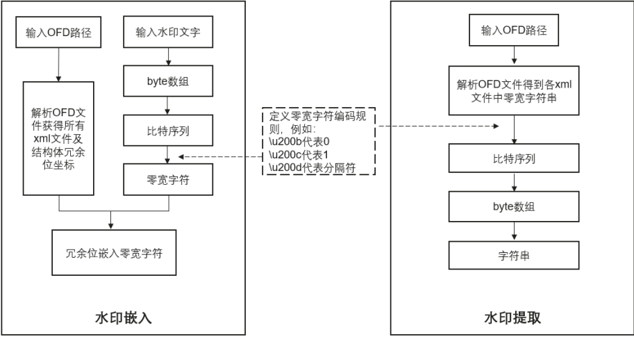
图 12 基于零宽字符的 OFD 隐式水印算法流程
