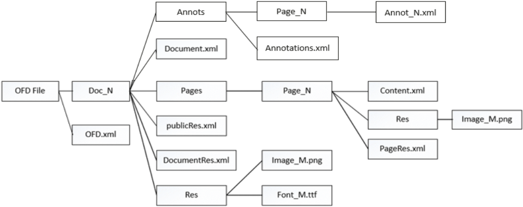
图 9 OFD 文件结构
