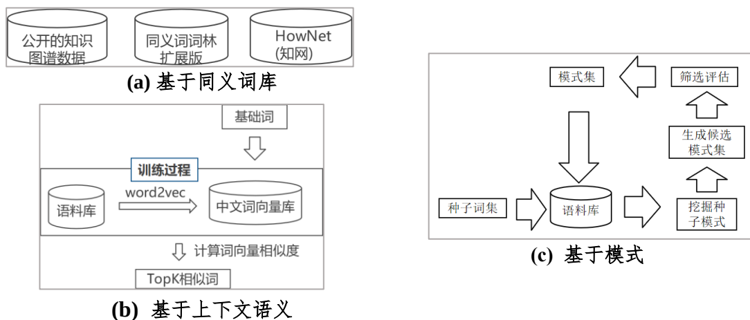
图 4 规则库自动增广方法
