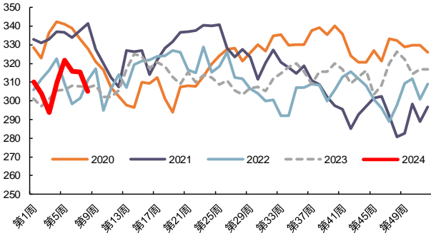
图 21: 热轧板卷周度产量 (万吨)
