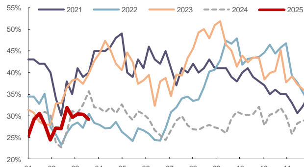
图 16: 沥青炼厂周开工率 (%)
