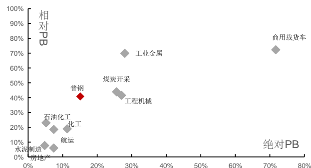
图 98：2013 年以来周期板块 PB 分位（横轴）与相对 PB 分位（纵轴）（%）
