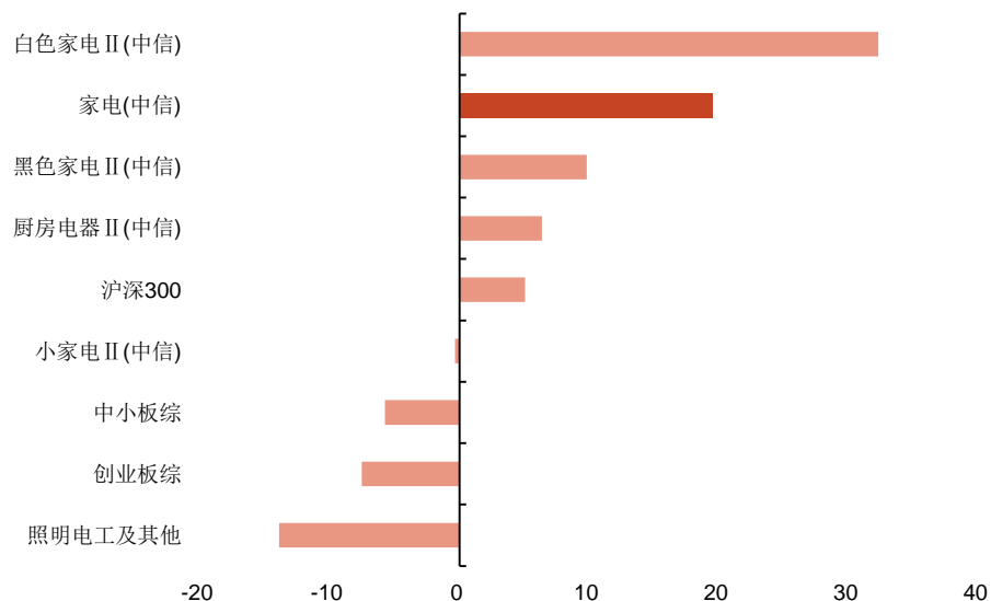
图1：中信家电细分行业24年至今涨跌幅（%）
