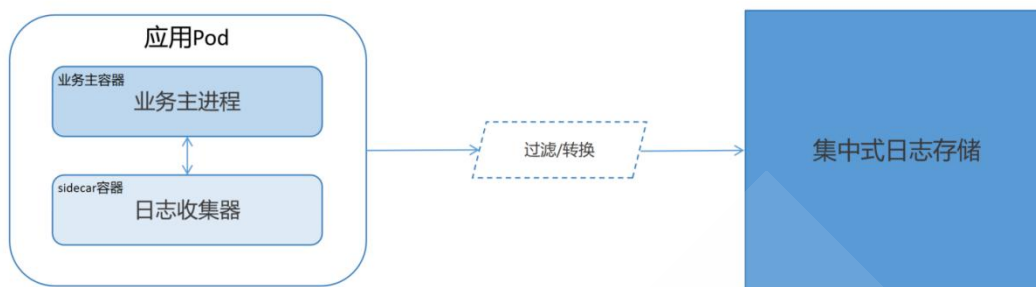
图 10: kubernetes 中常见日志收集方式
