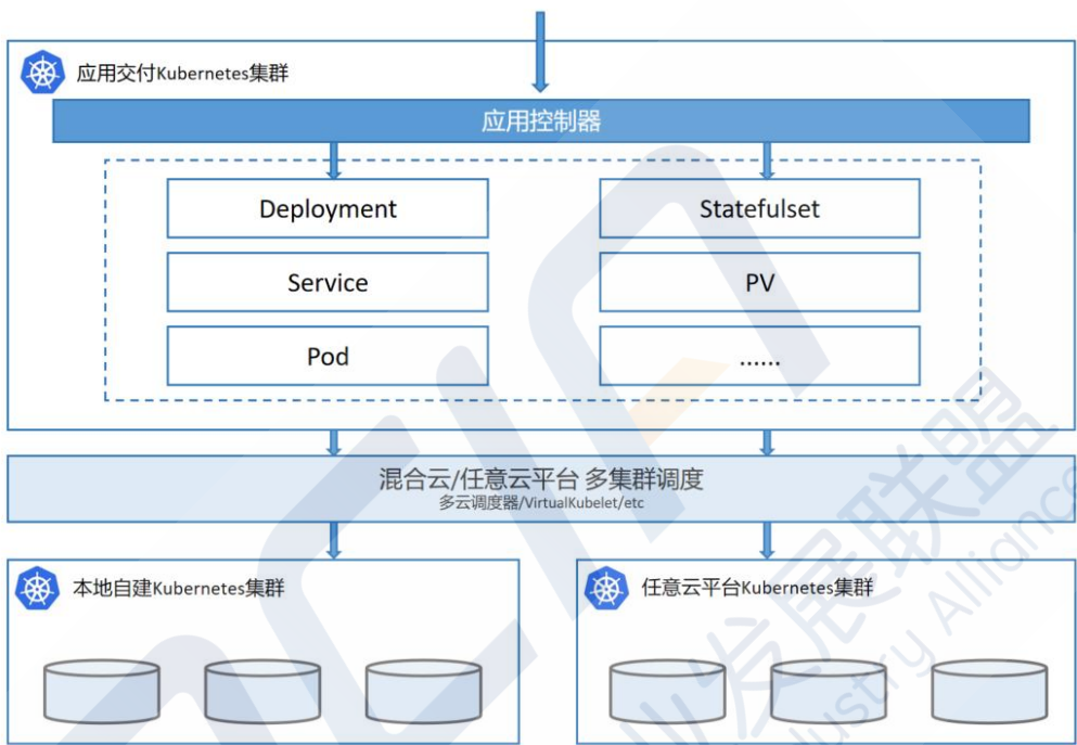
图 20：多云/混合云部署示意图
