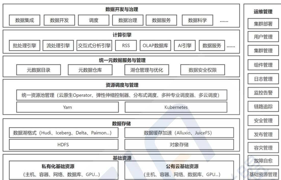
图 22：云原生湖仓一体数据平台参考架构
