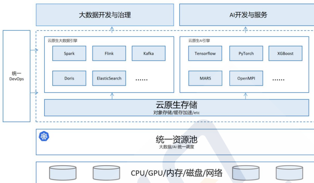
图 21：大数据/AI 混合部署
