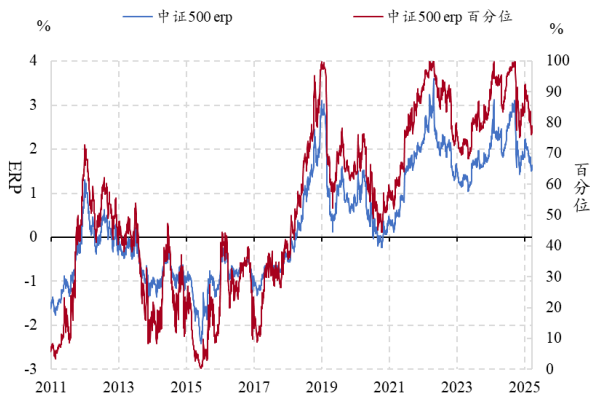
图表 33. 中证 500 指数 erp 及百分位
