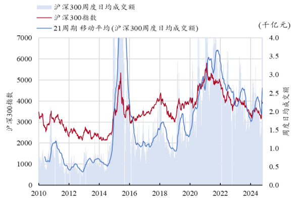
图表 22 沪深 300 指数表现及日均成交额
